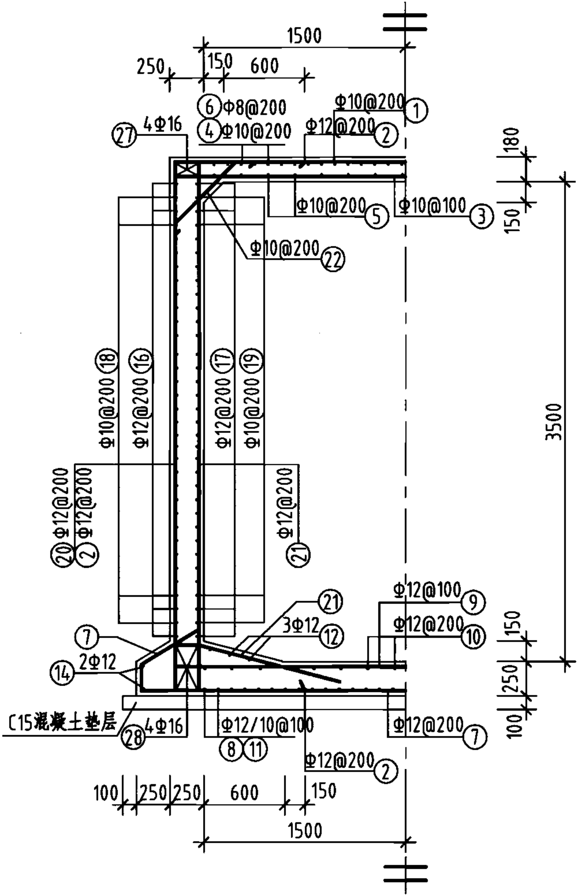
2-2 剖面图
