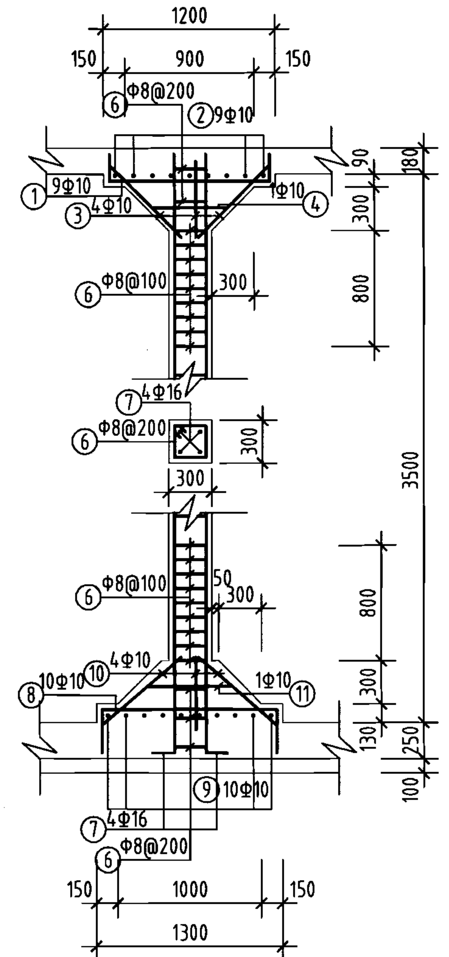
支柱配筋
