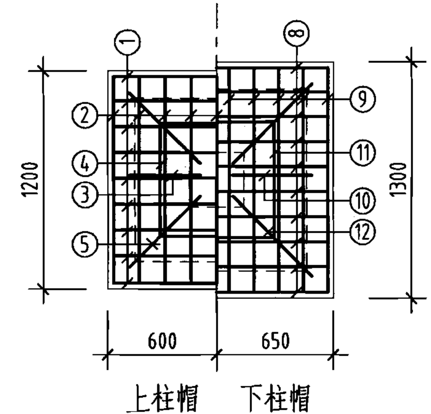
柱帽配筋
