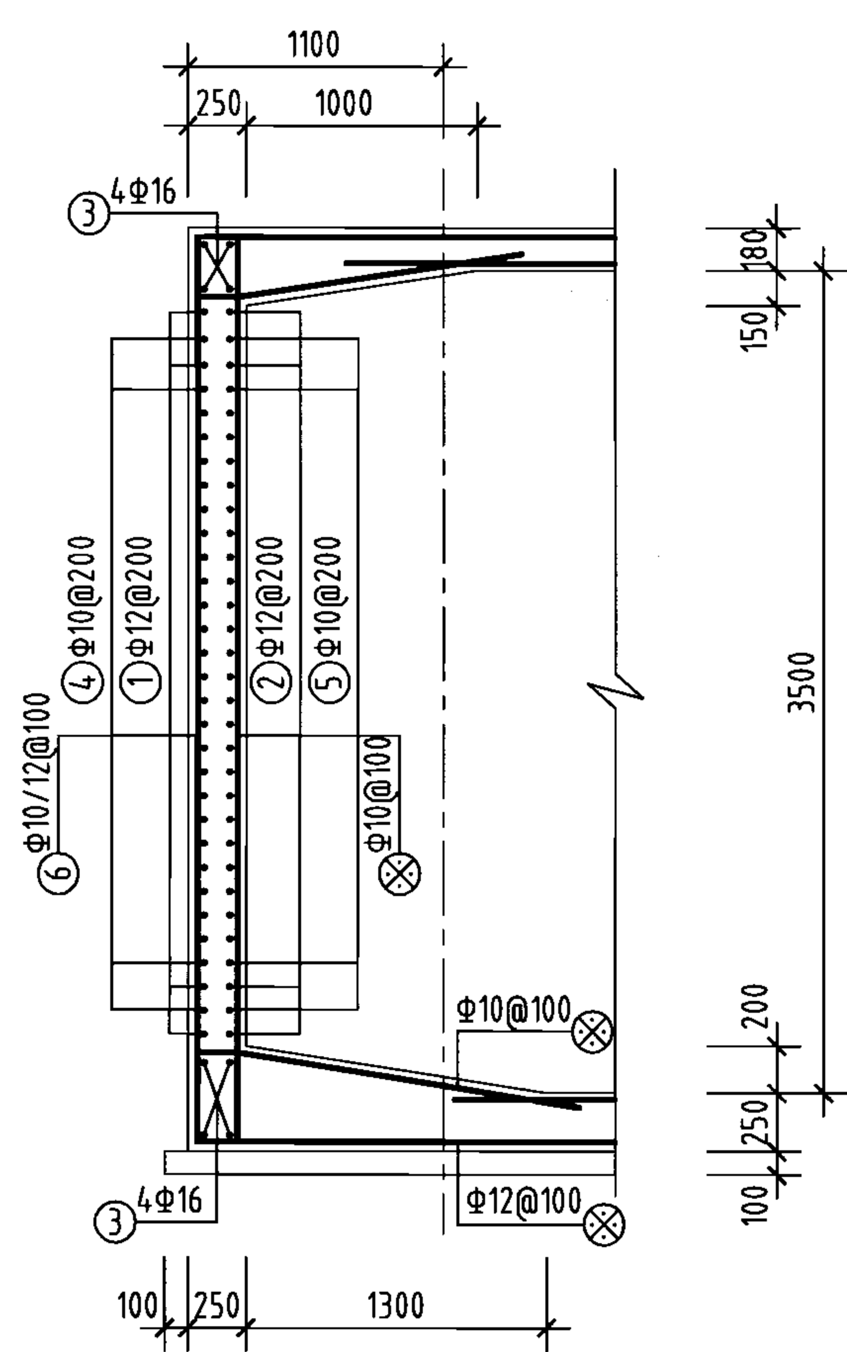
1-1剖面
