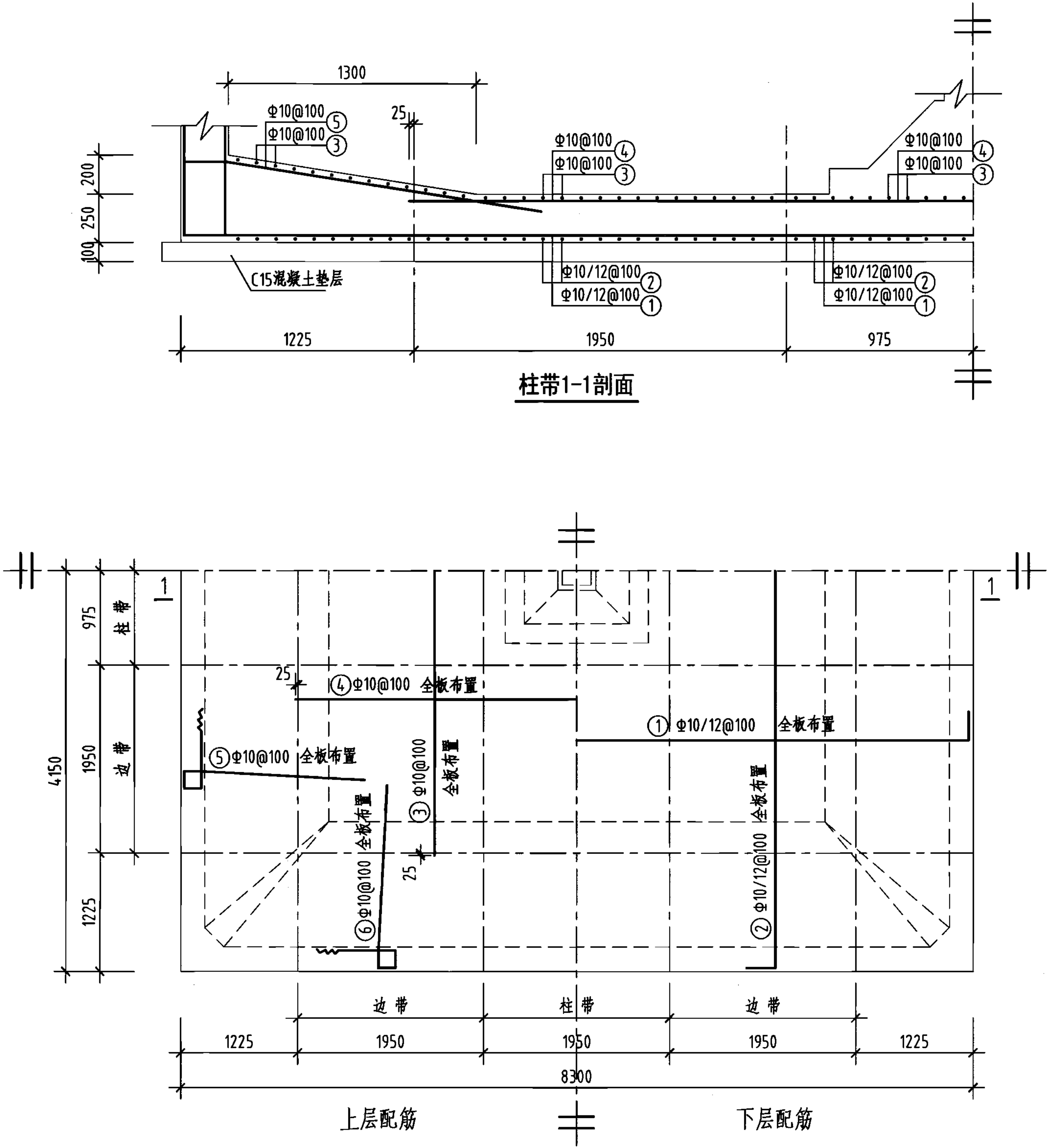
底板平面配筋图
