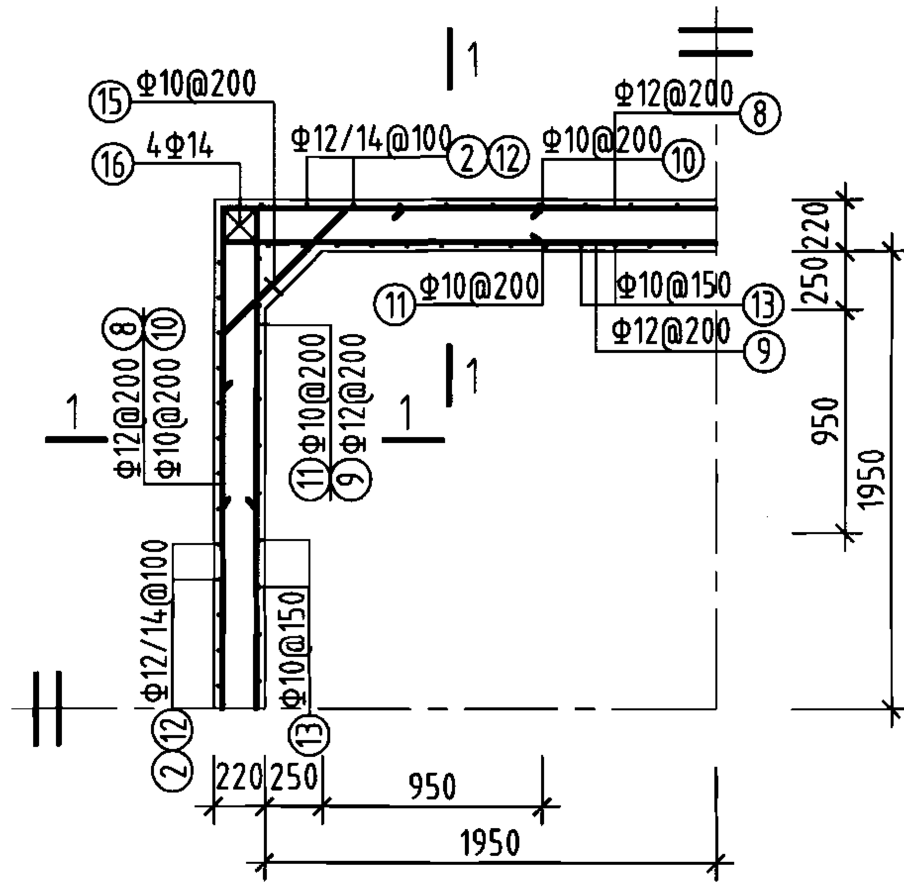
池壁平面配筋图
