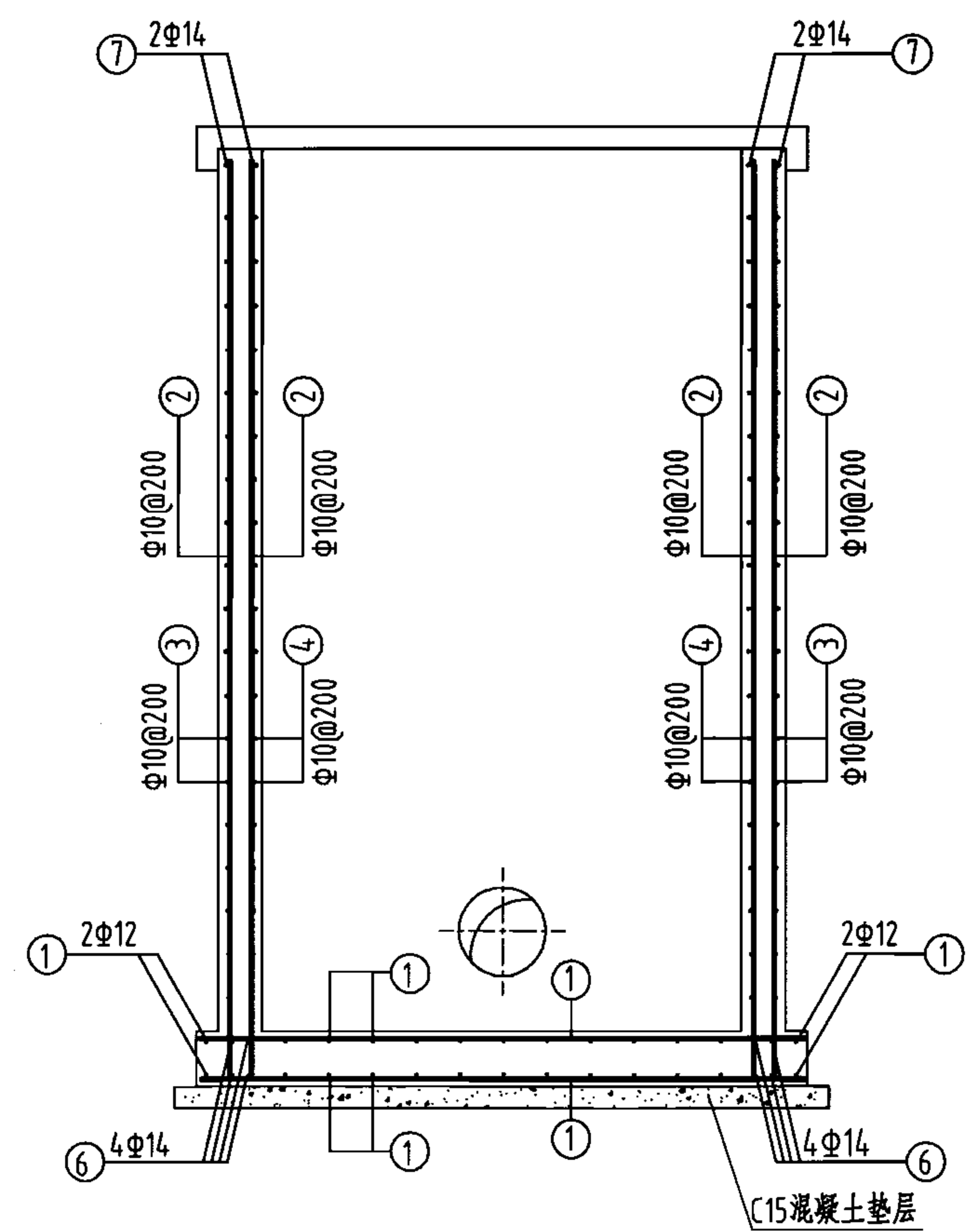
2-2 剖面图
