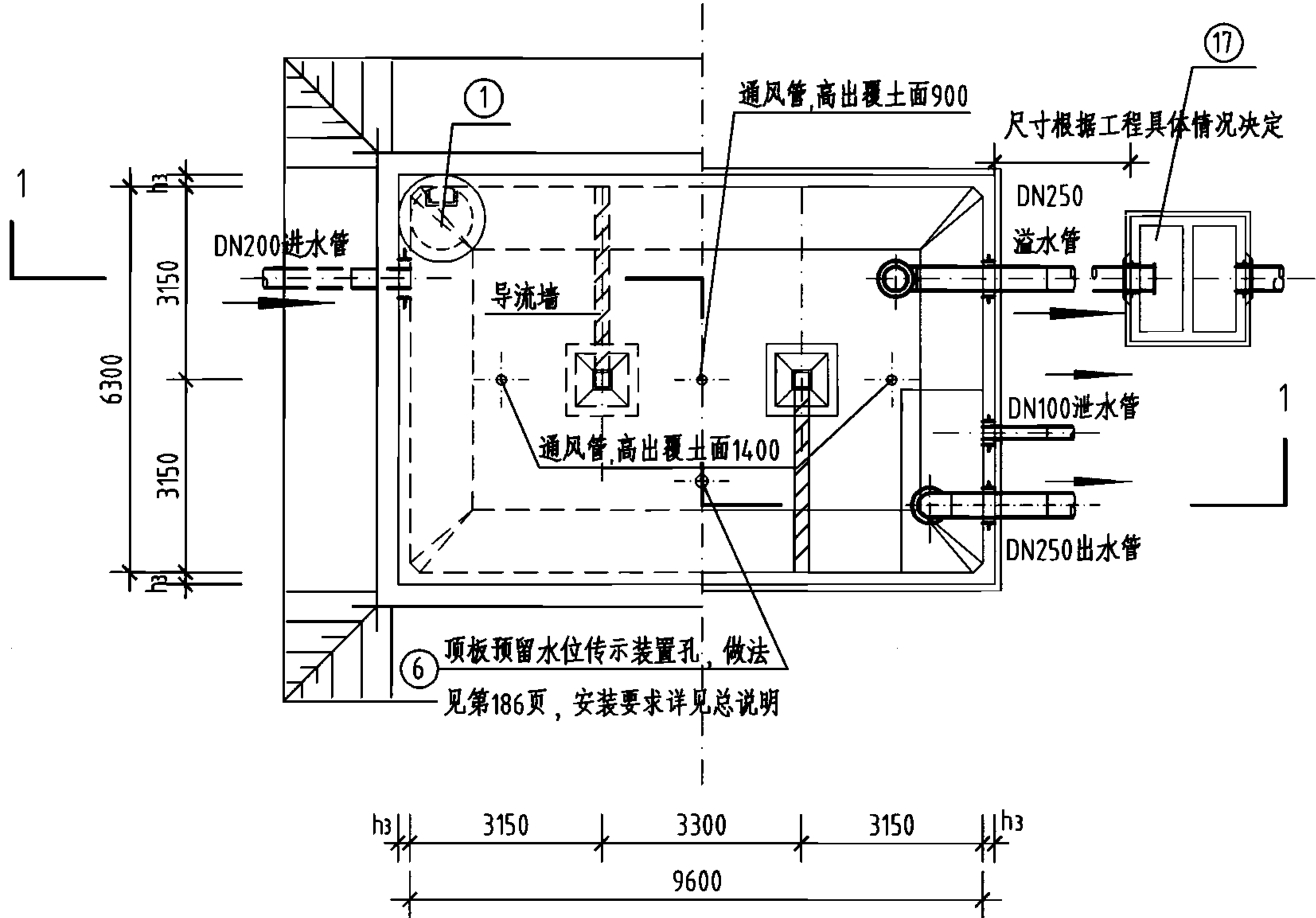
平面图
