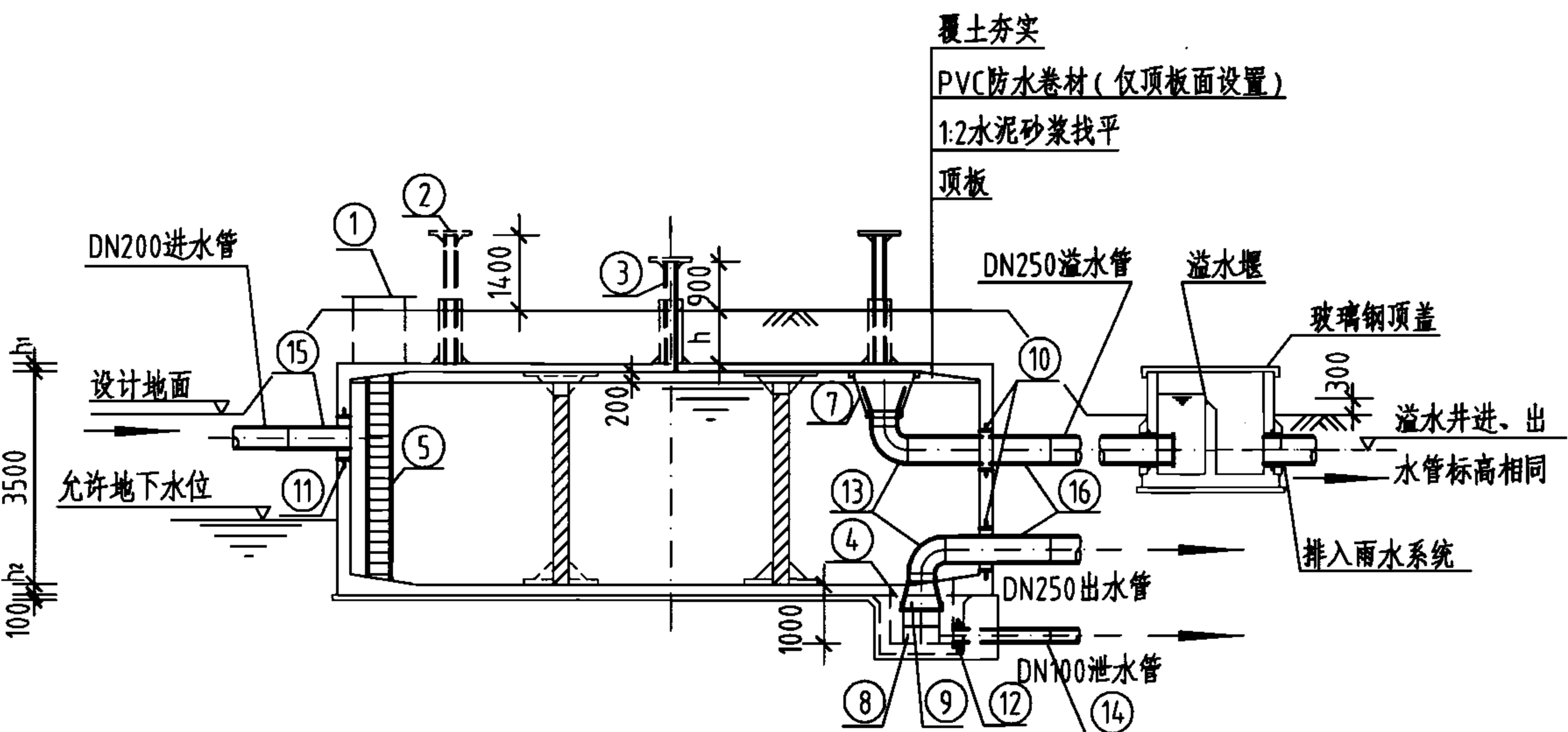
1-1剖面图
