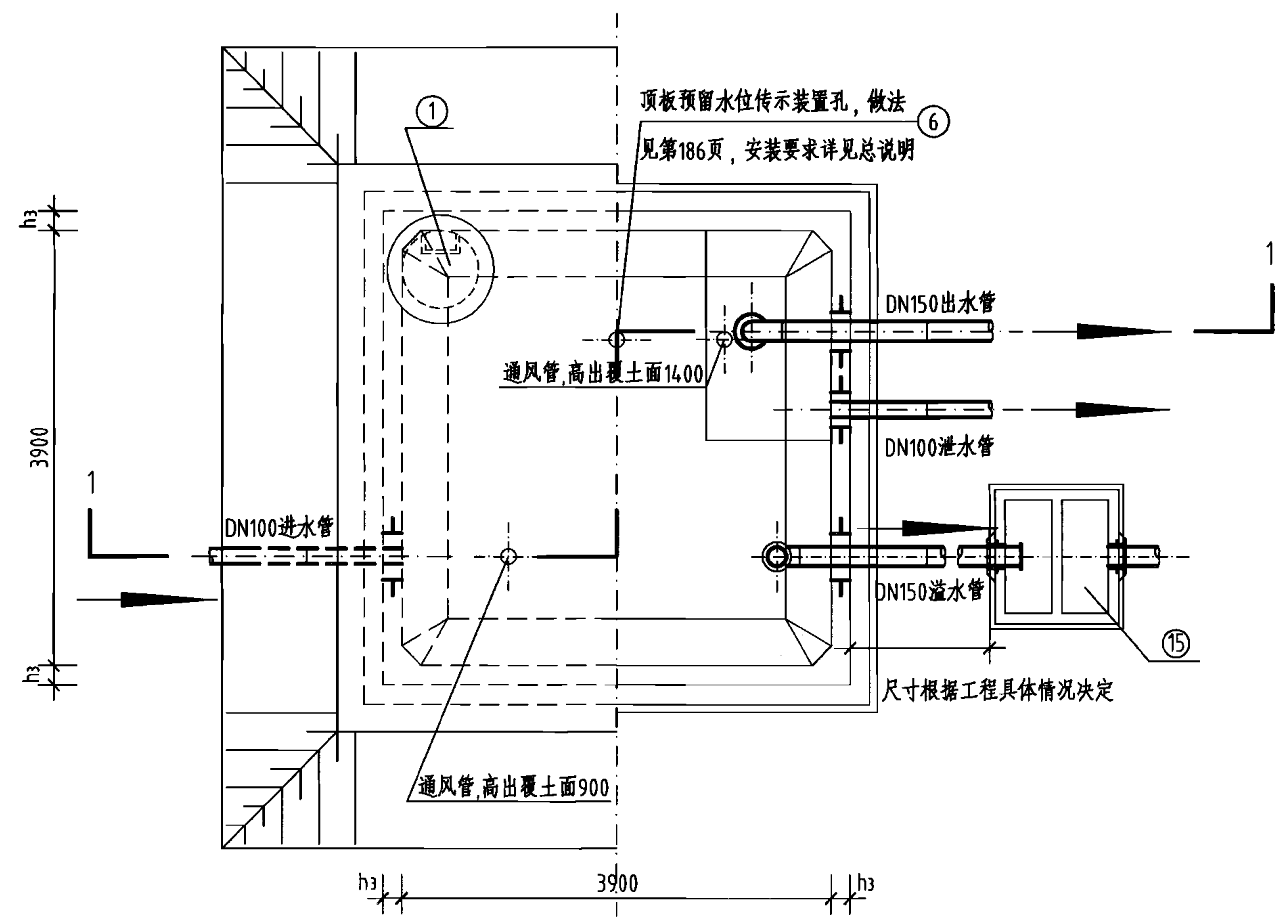
平面图
