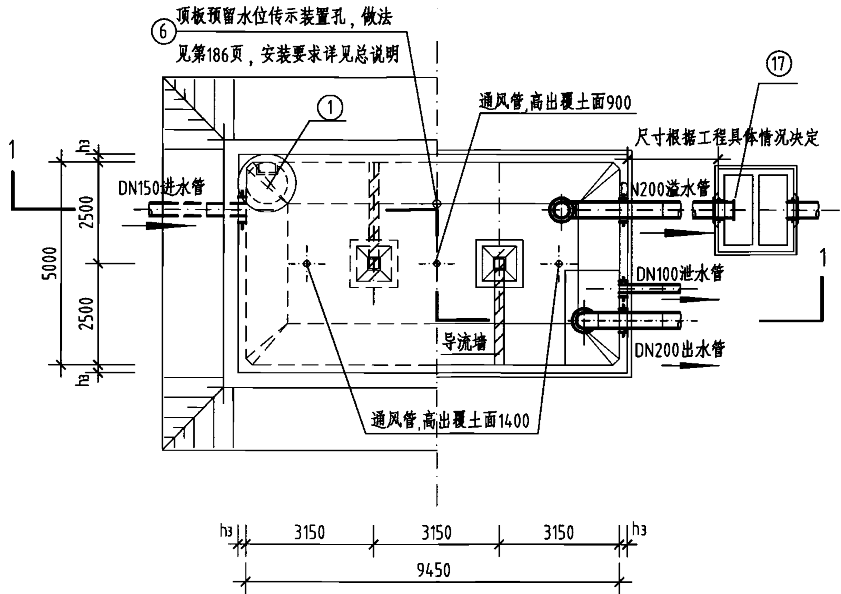
平面图
