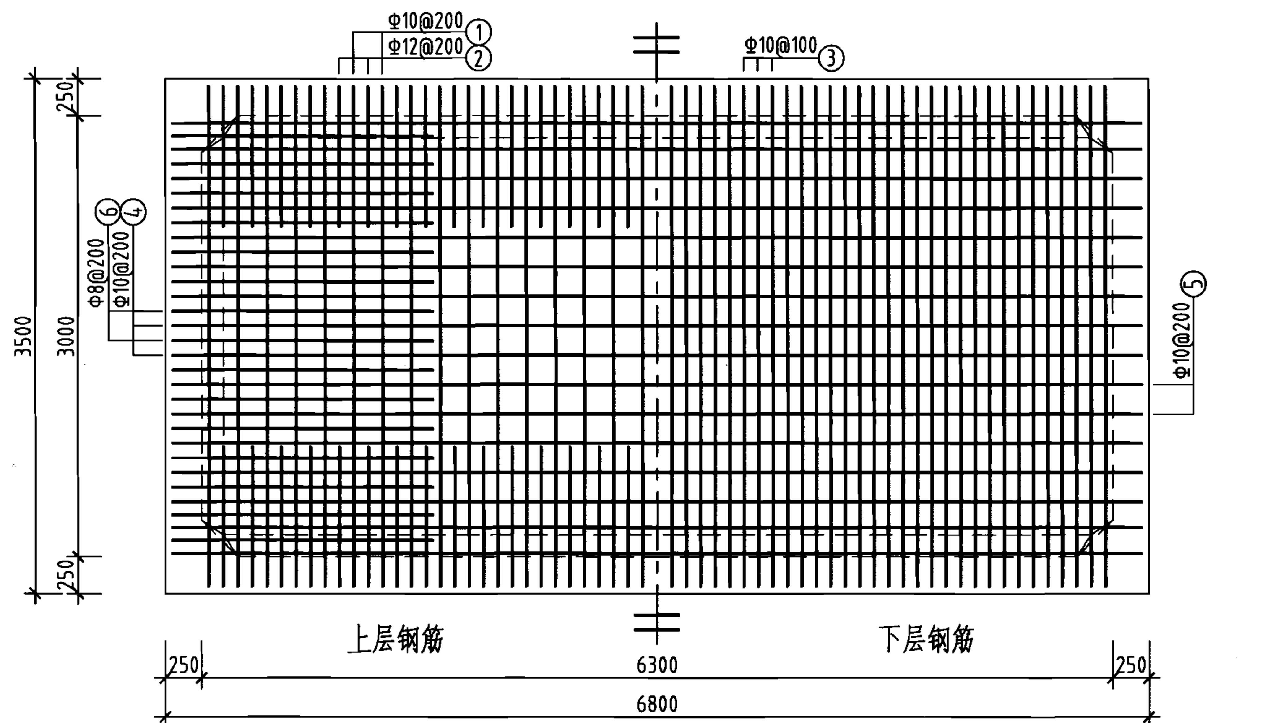
池顶板配筋图
