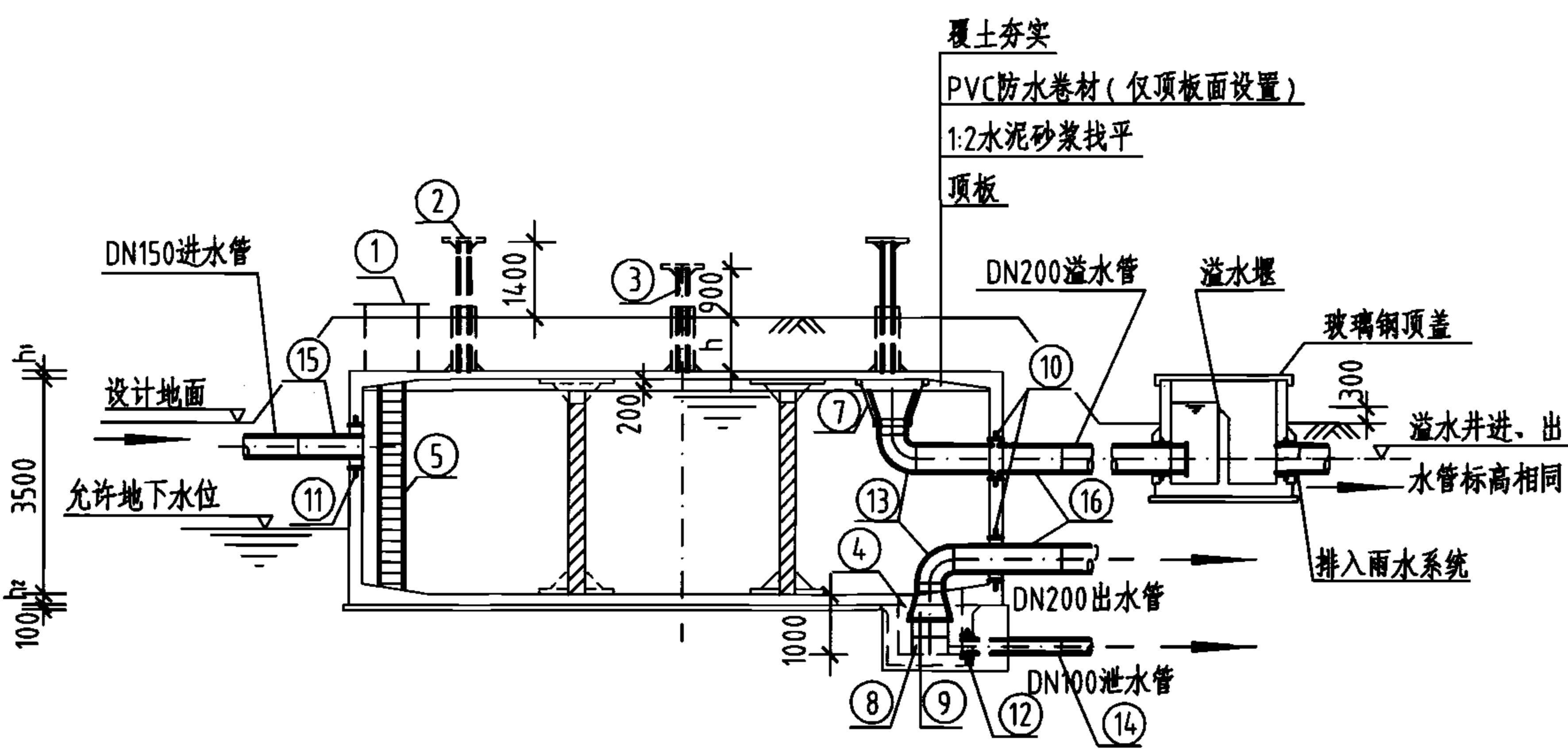
1-1剖面图
