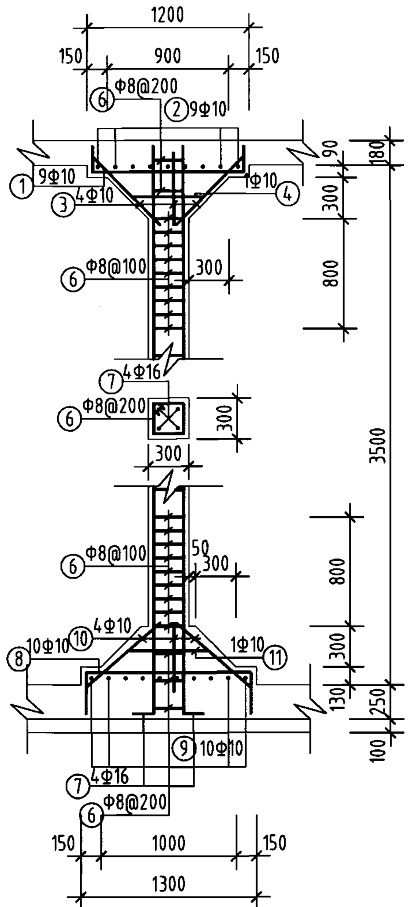
支柱配筋
