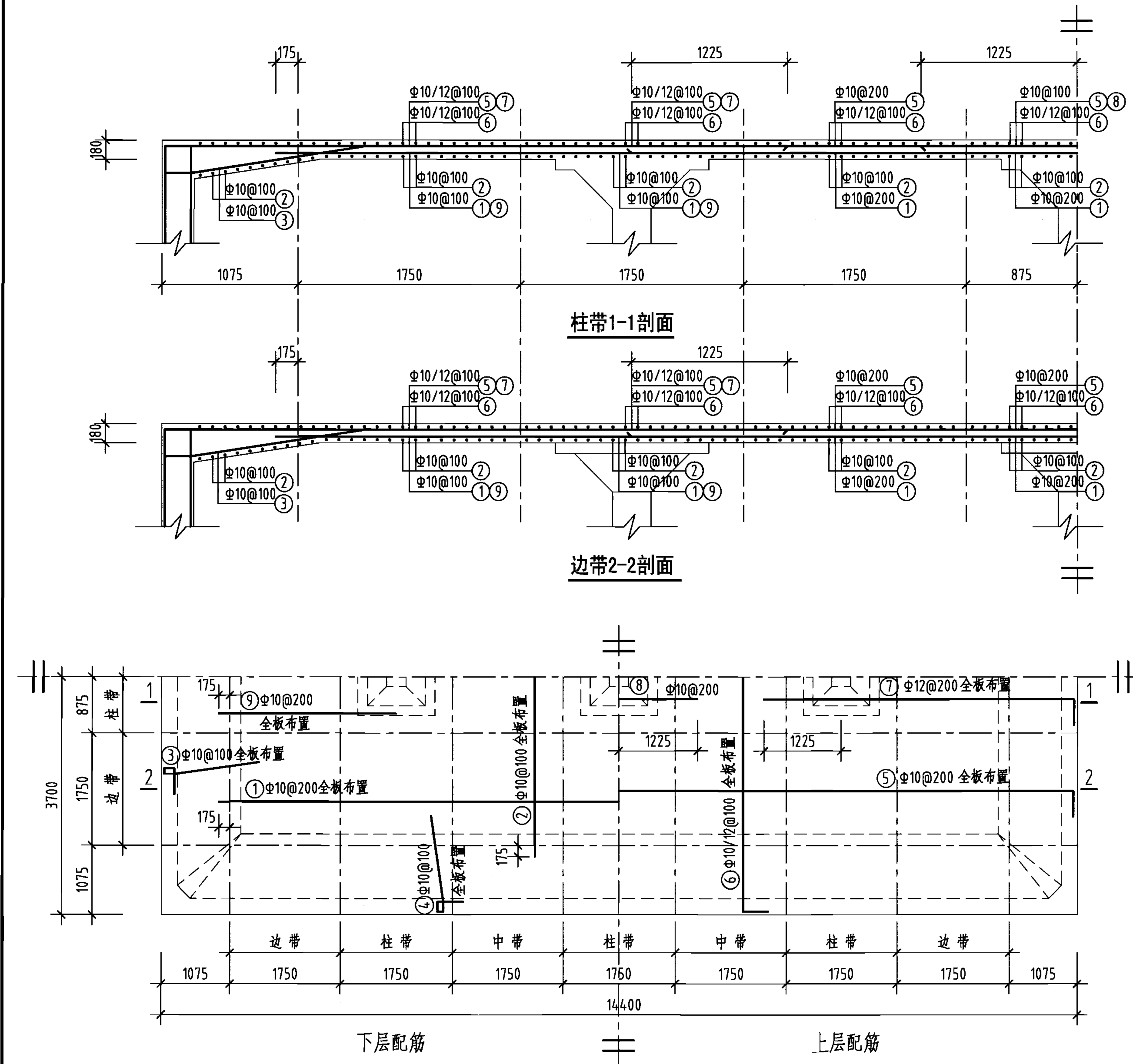
顶板平面配筋图
