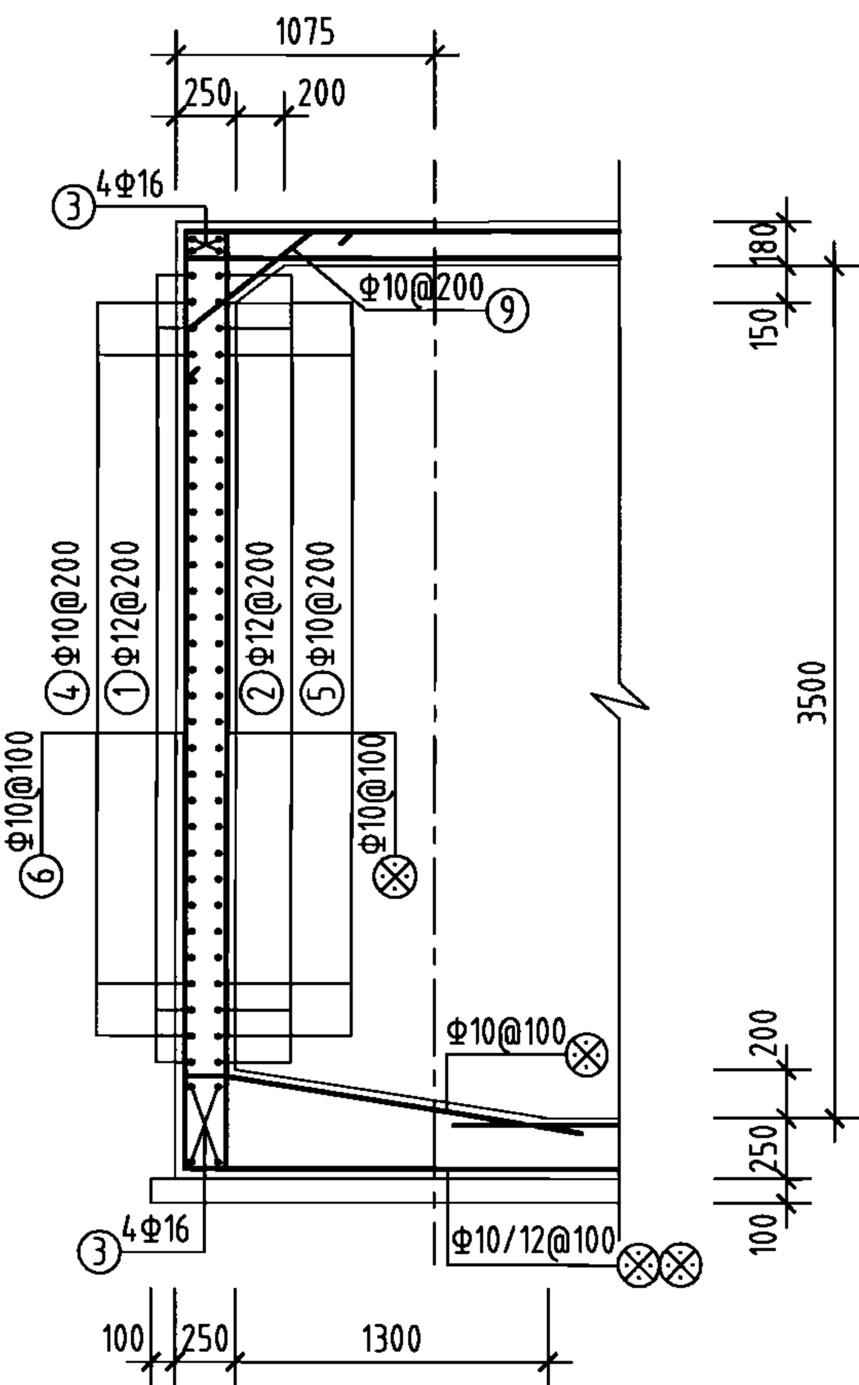
1-1剖面 (1'-1'剖面)
