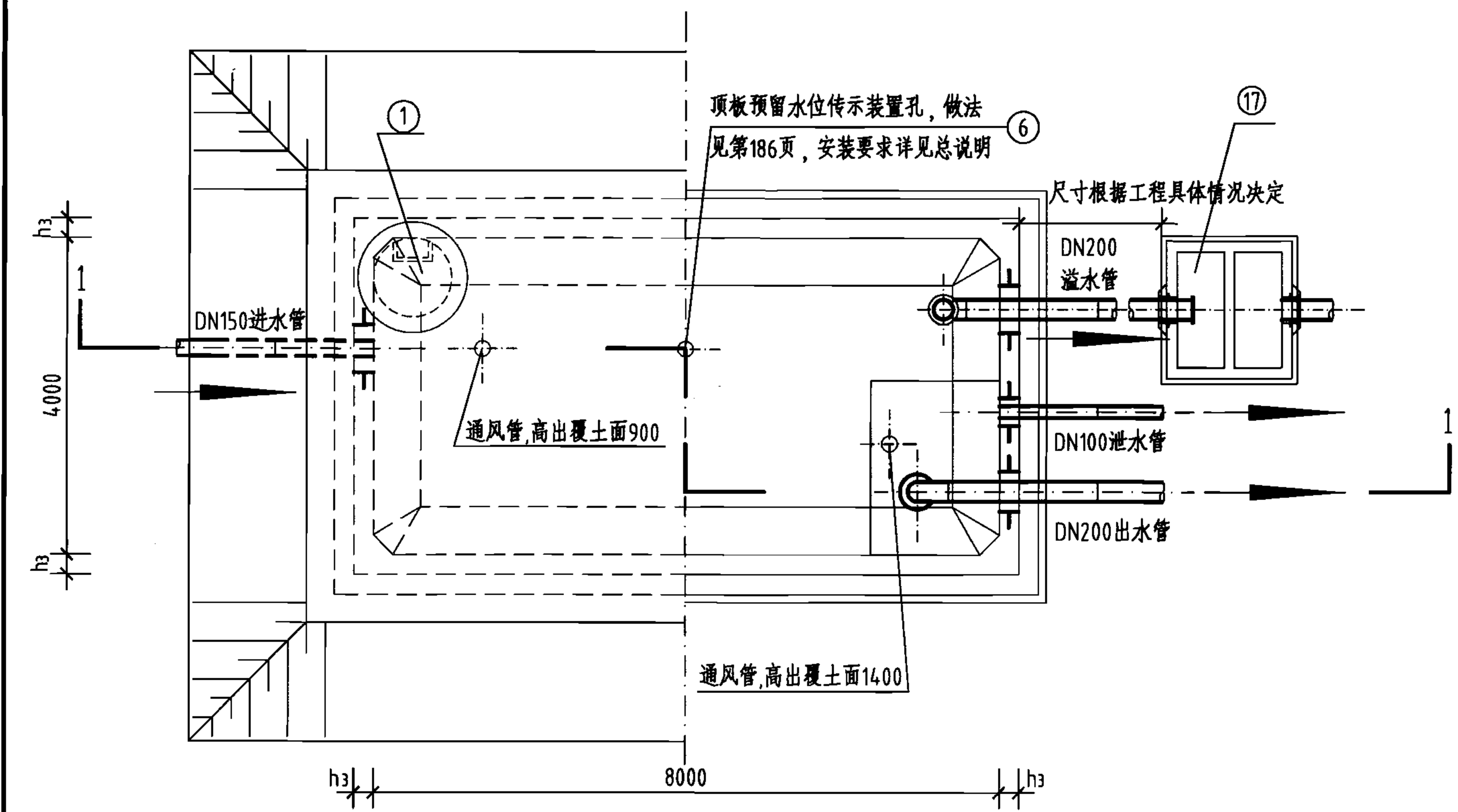
平面图
