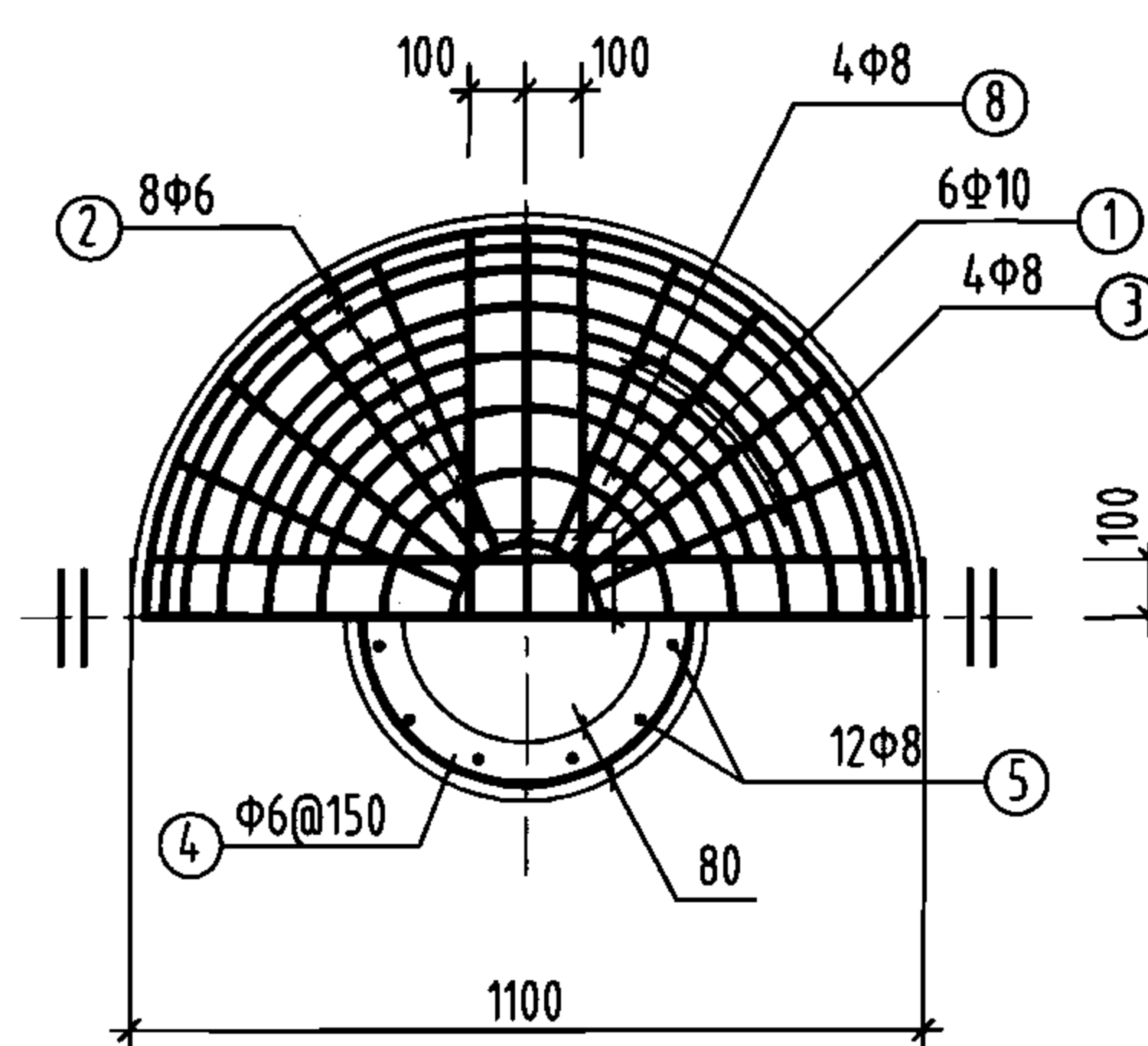
通风管、帽配筋图
