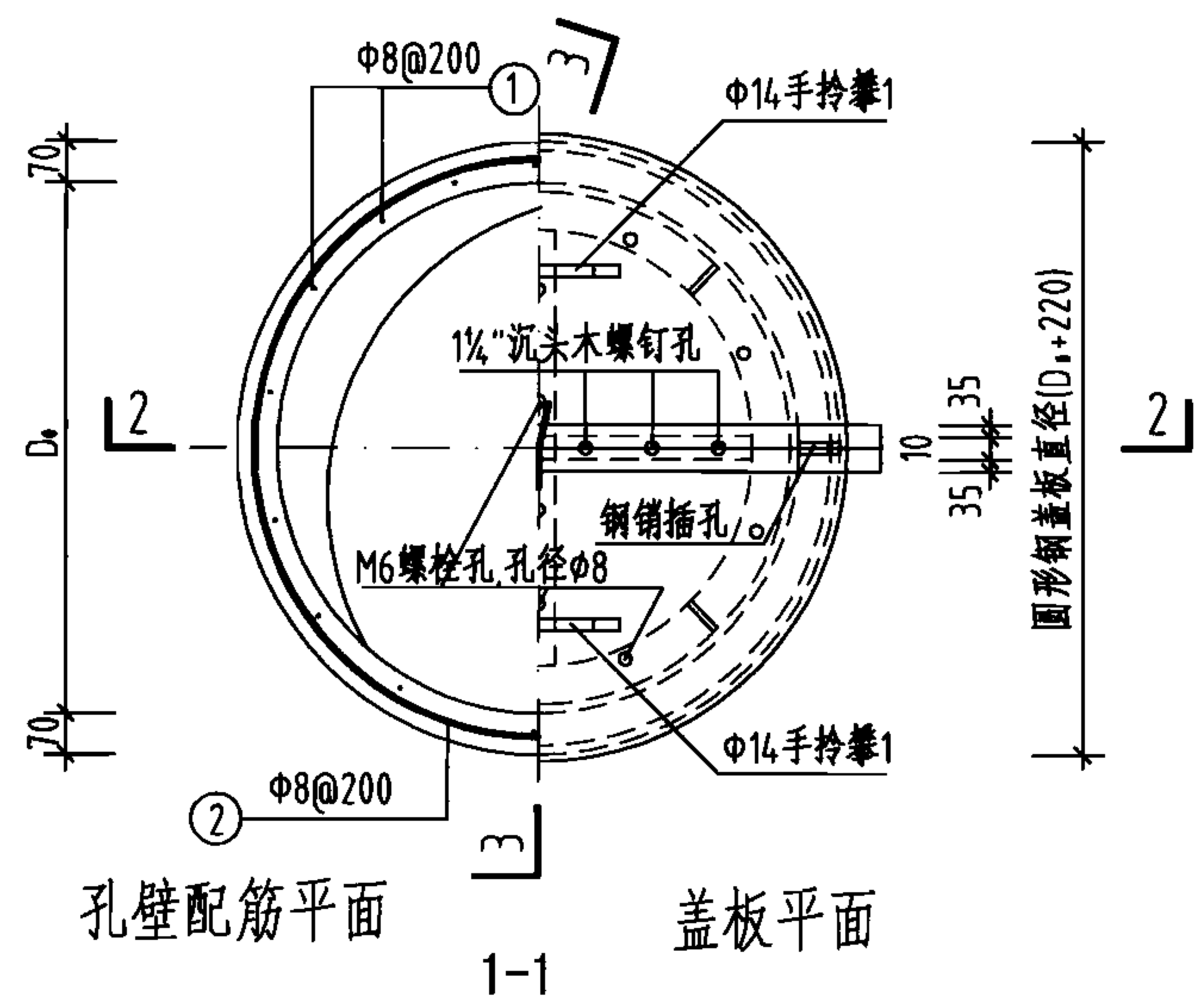
检修孔钢筋布置图
