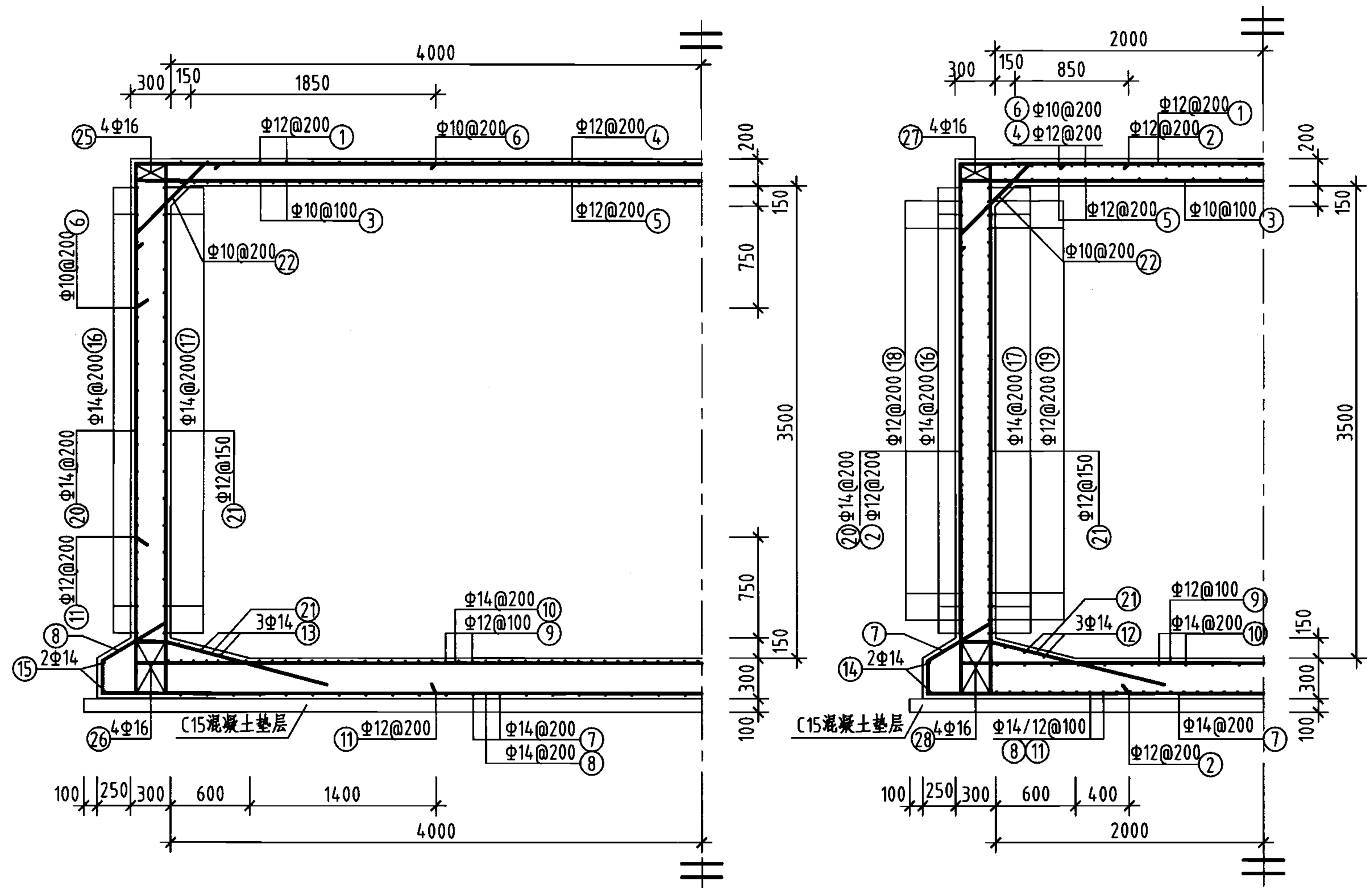
1-1 剖面图
