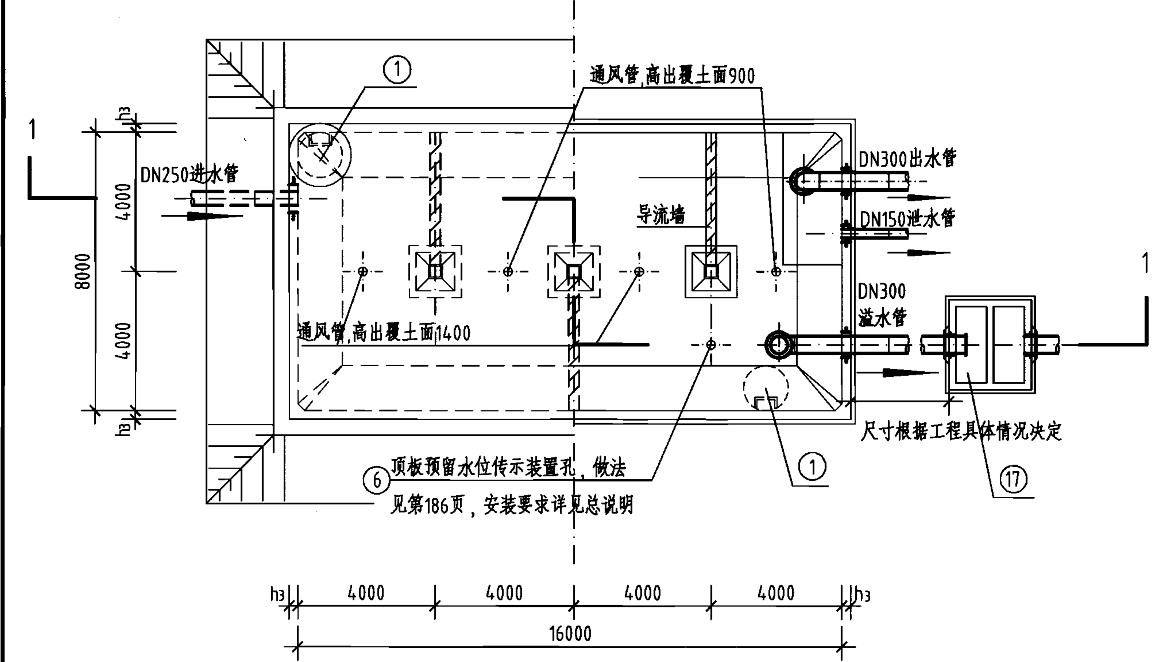
平面图
