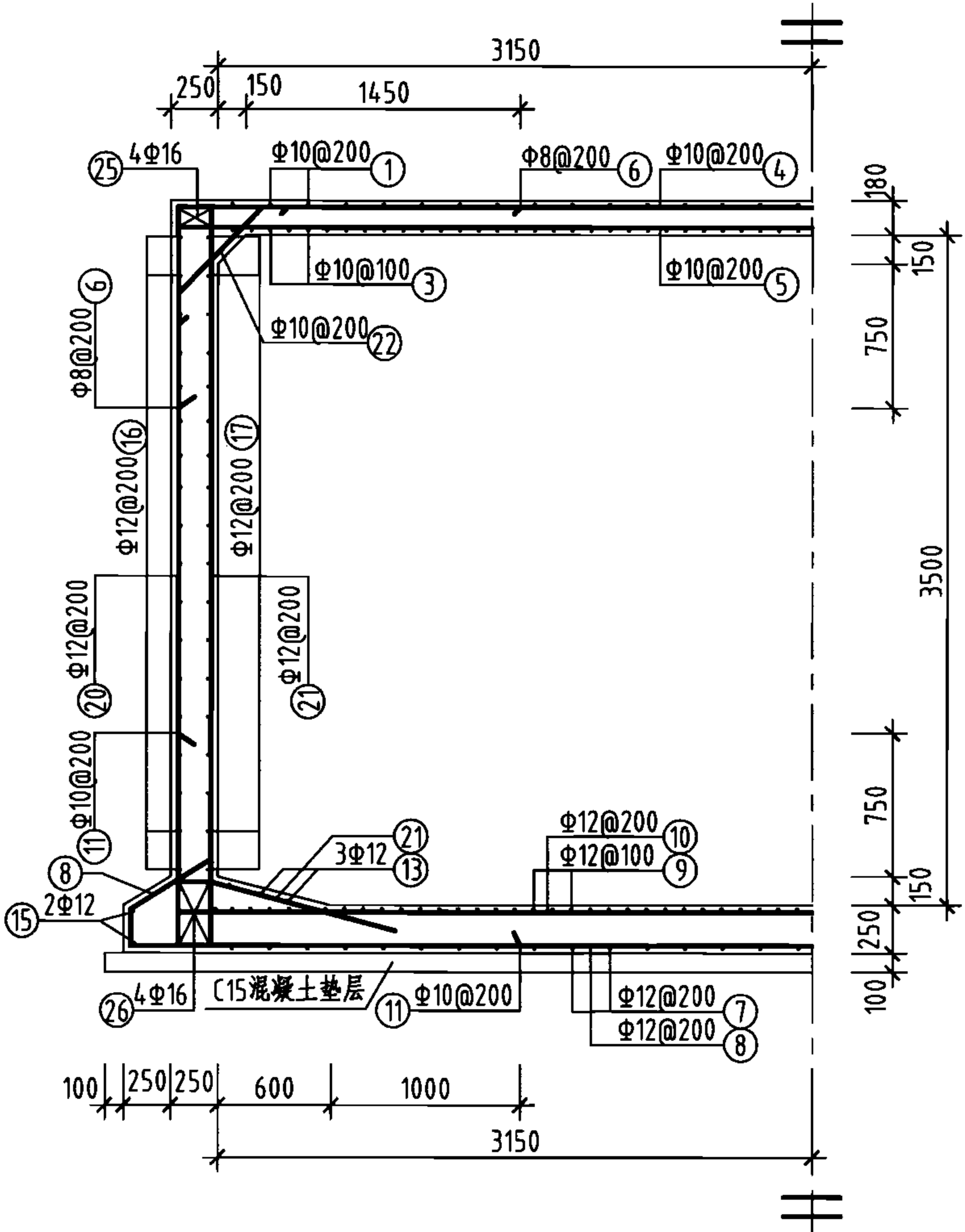
1-1 剖面图
