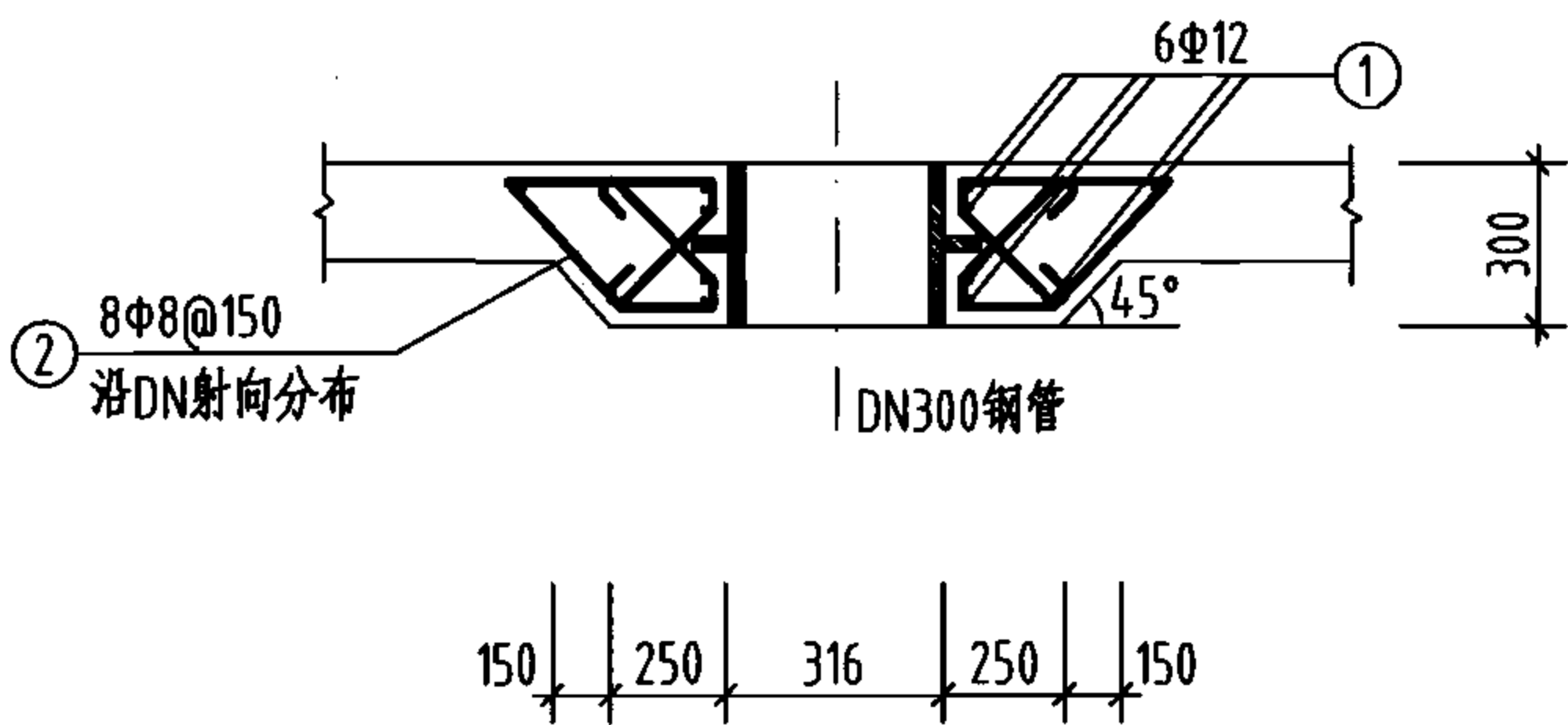
1-1剖面图
