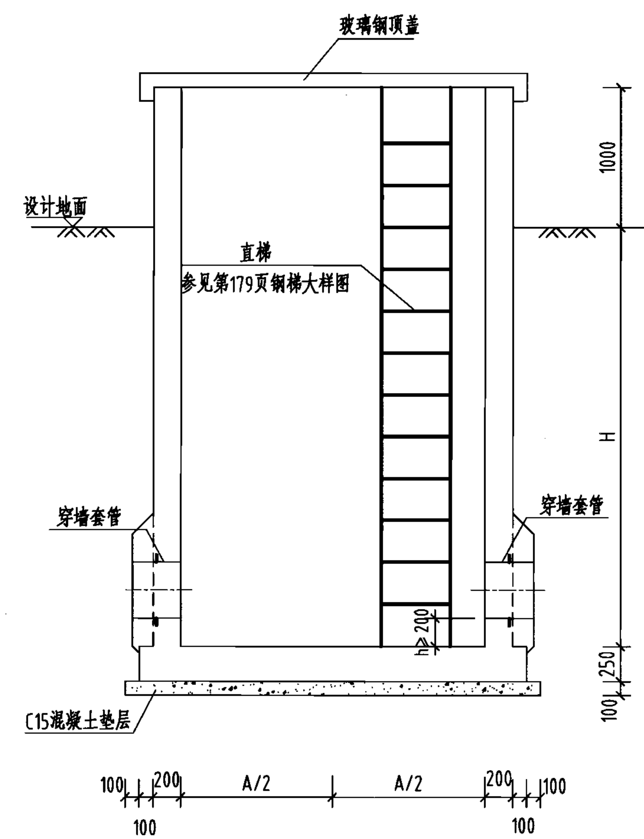
1-1 剖面图
