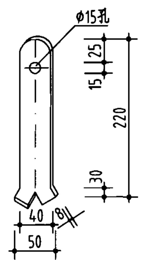
钢销
