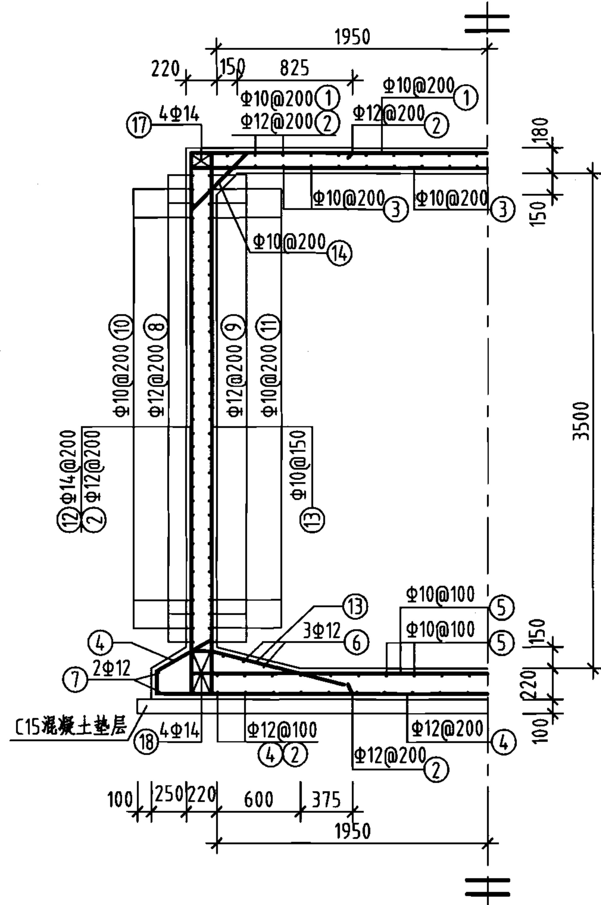
1-1 剖面图
