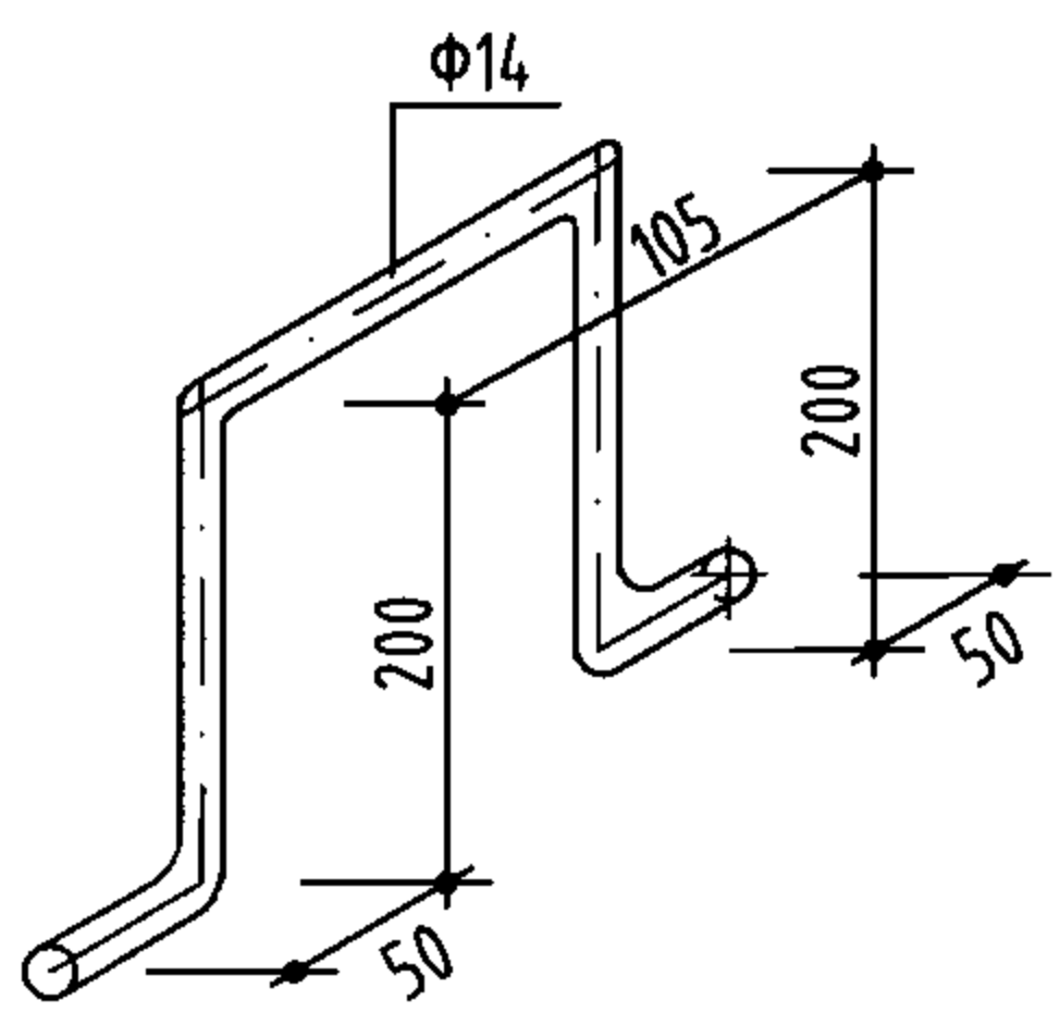
钢扣攀2
