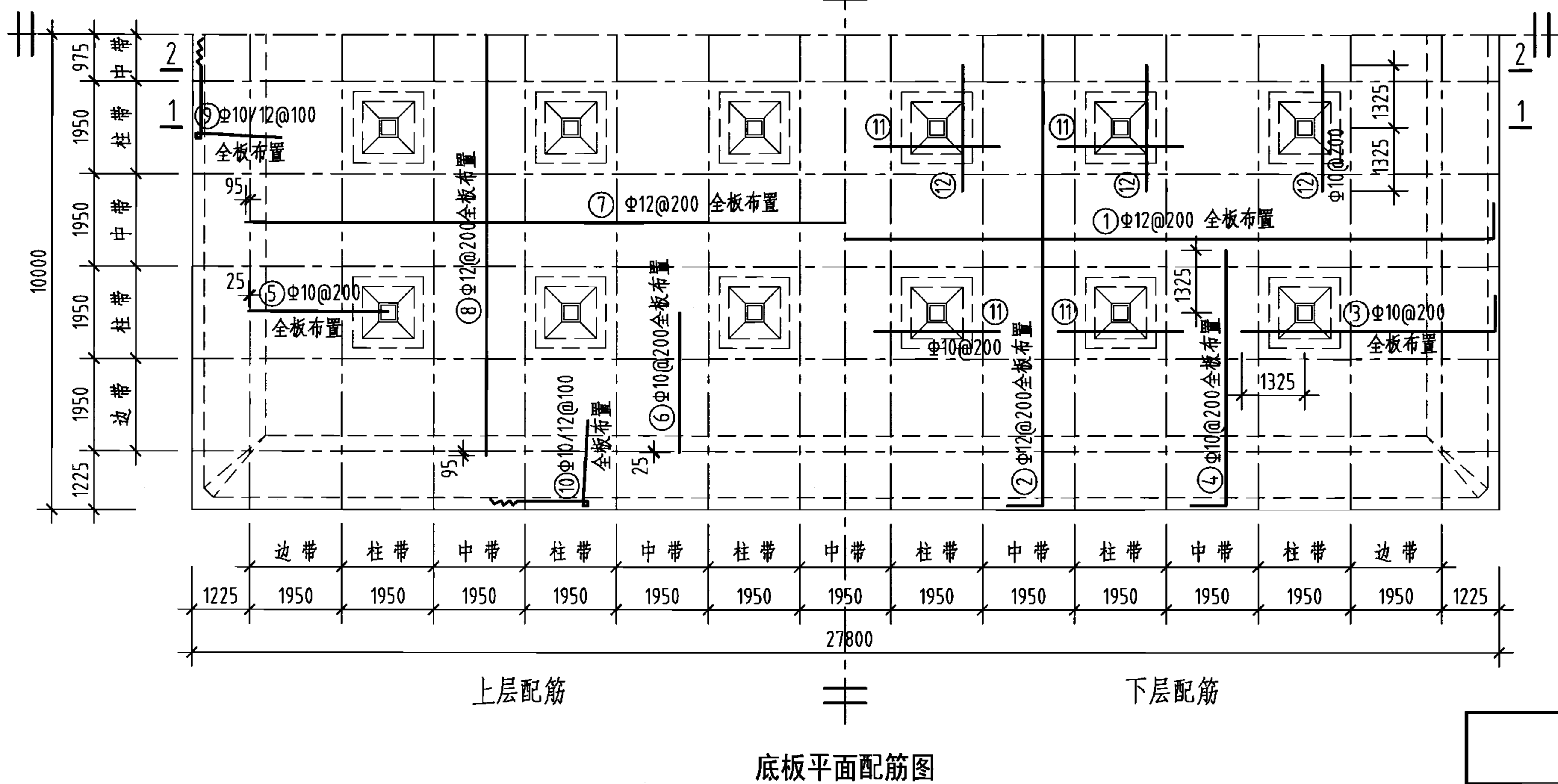
2000m 3 矩形蓄水池底板配筋图 (池顶覆土500mm)
