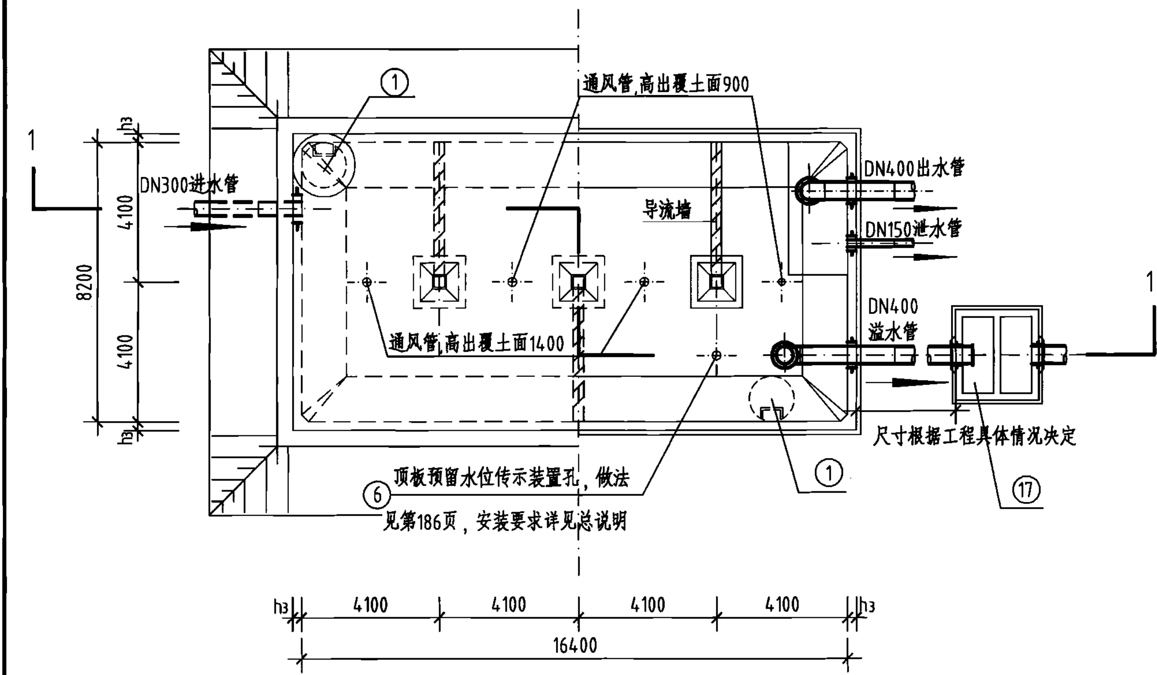
平面图
