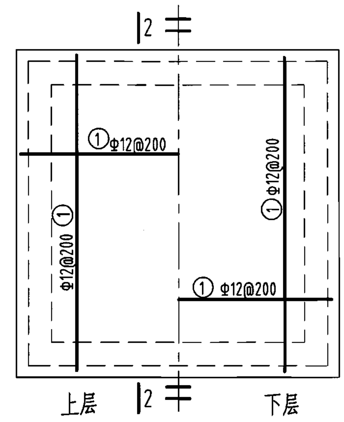
底板配筋
