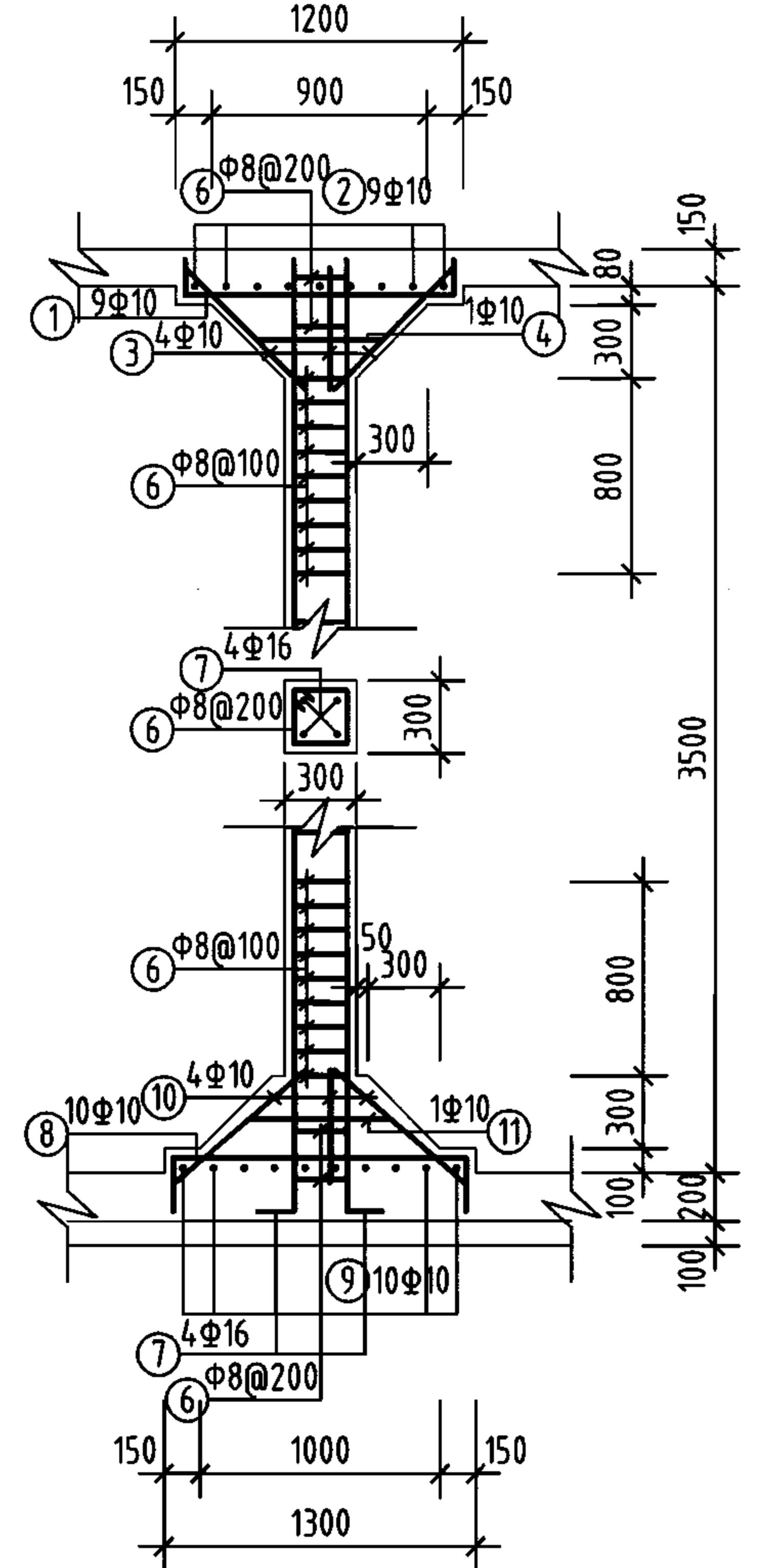
支柱配筋
