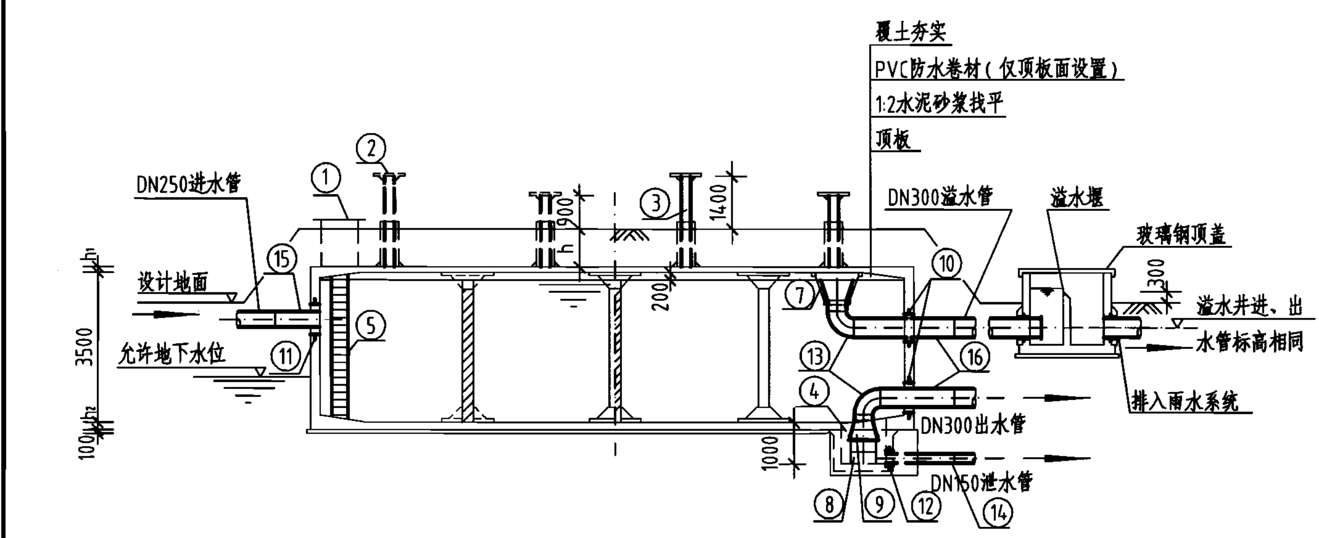
1-1剖面图
