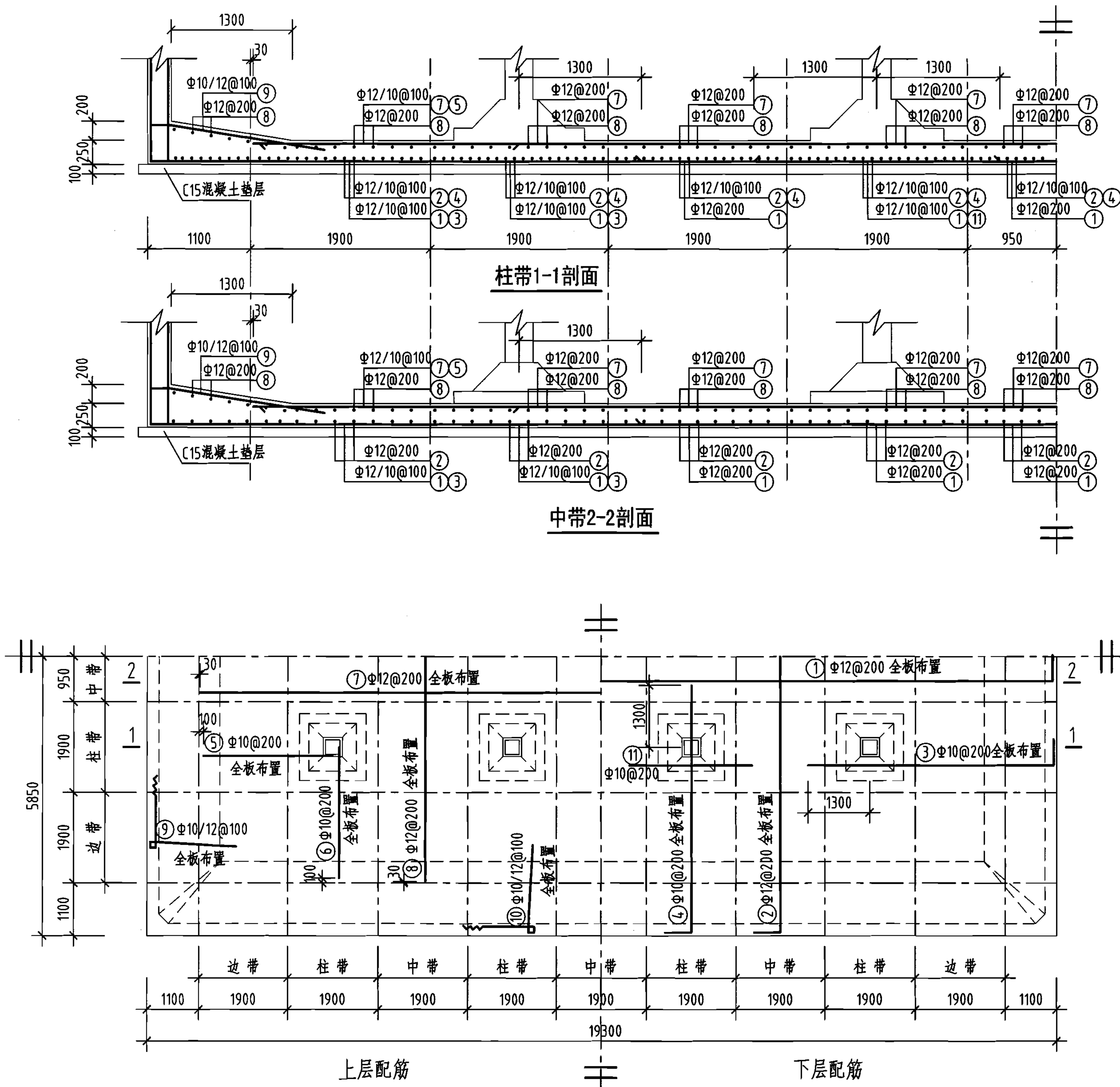
底板平面配筋图
