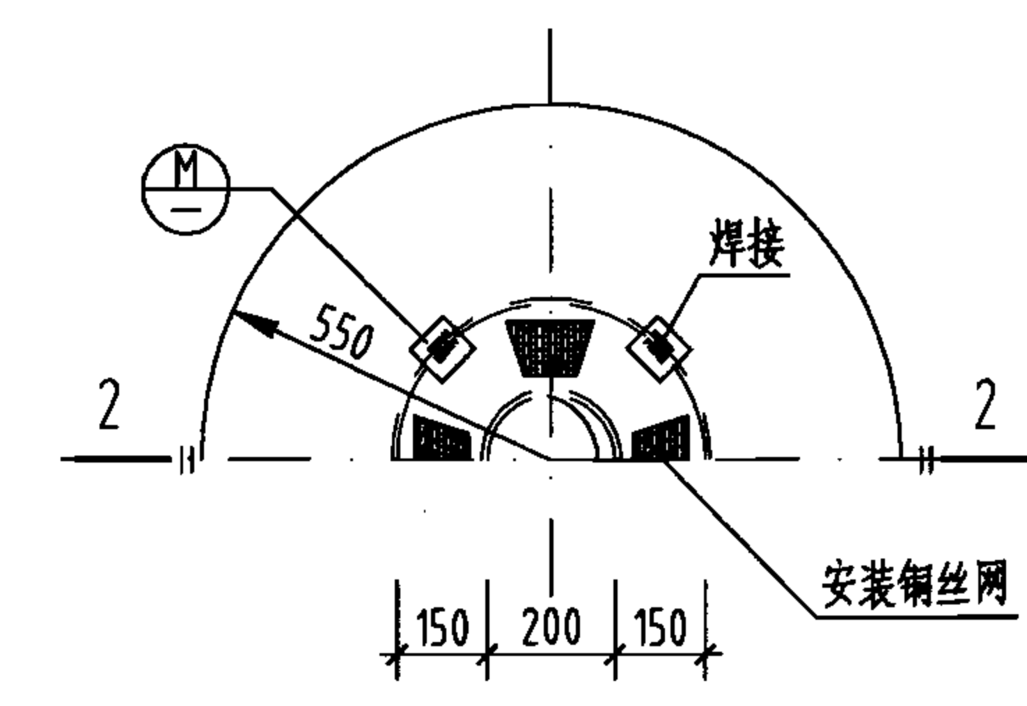
A型通风管、帽平面
