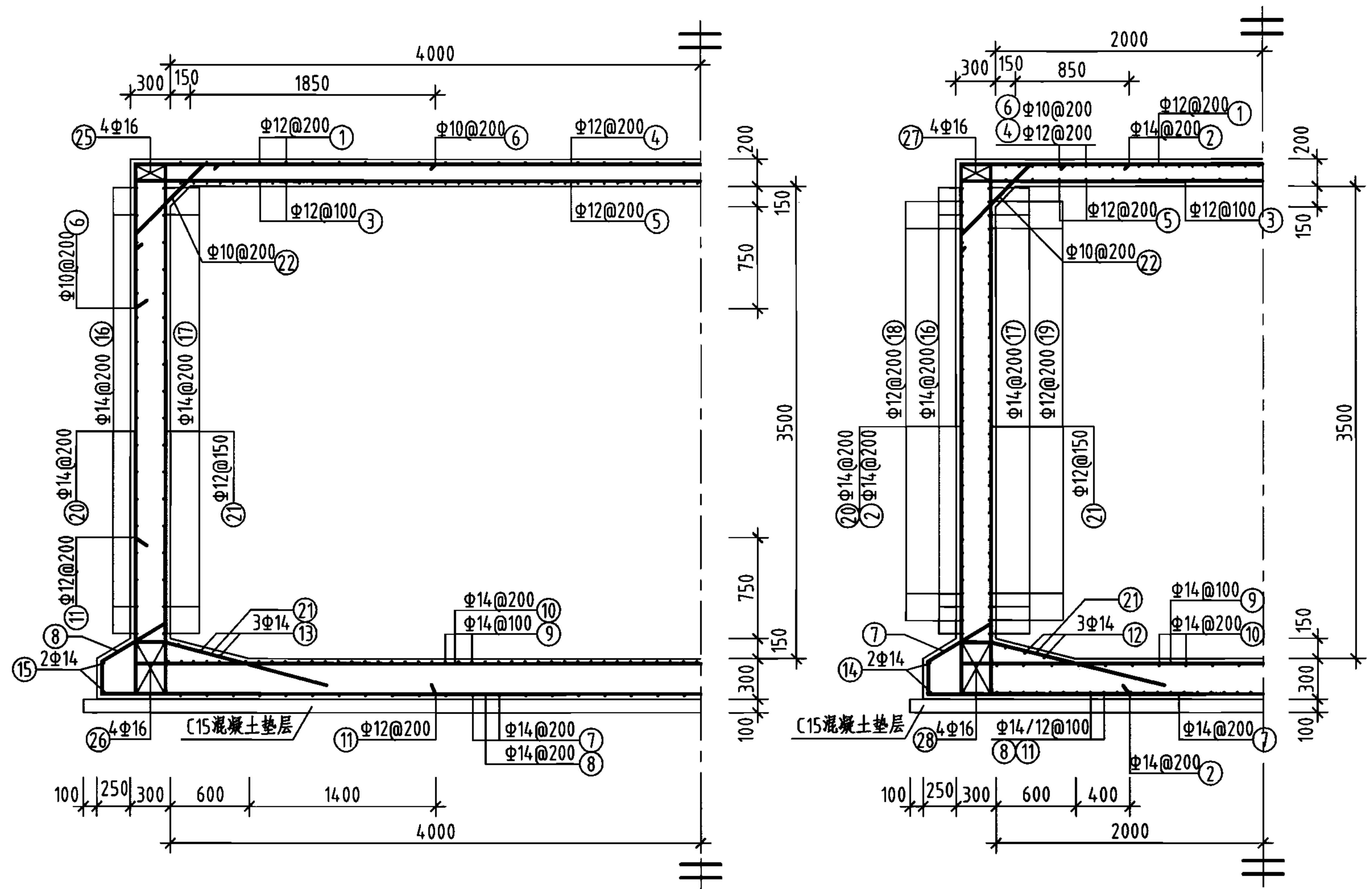
1-1 剖面图
