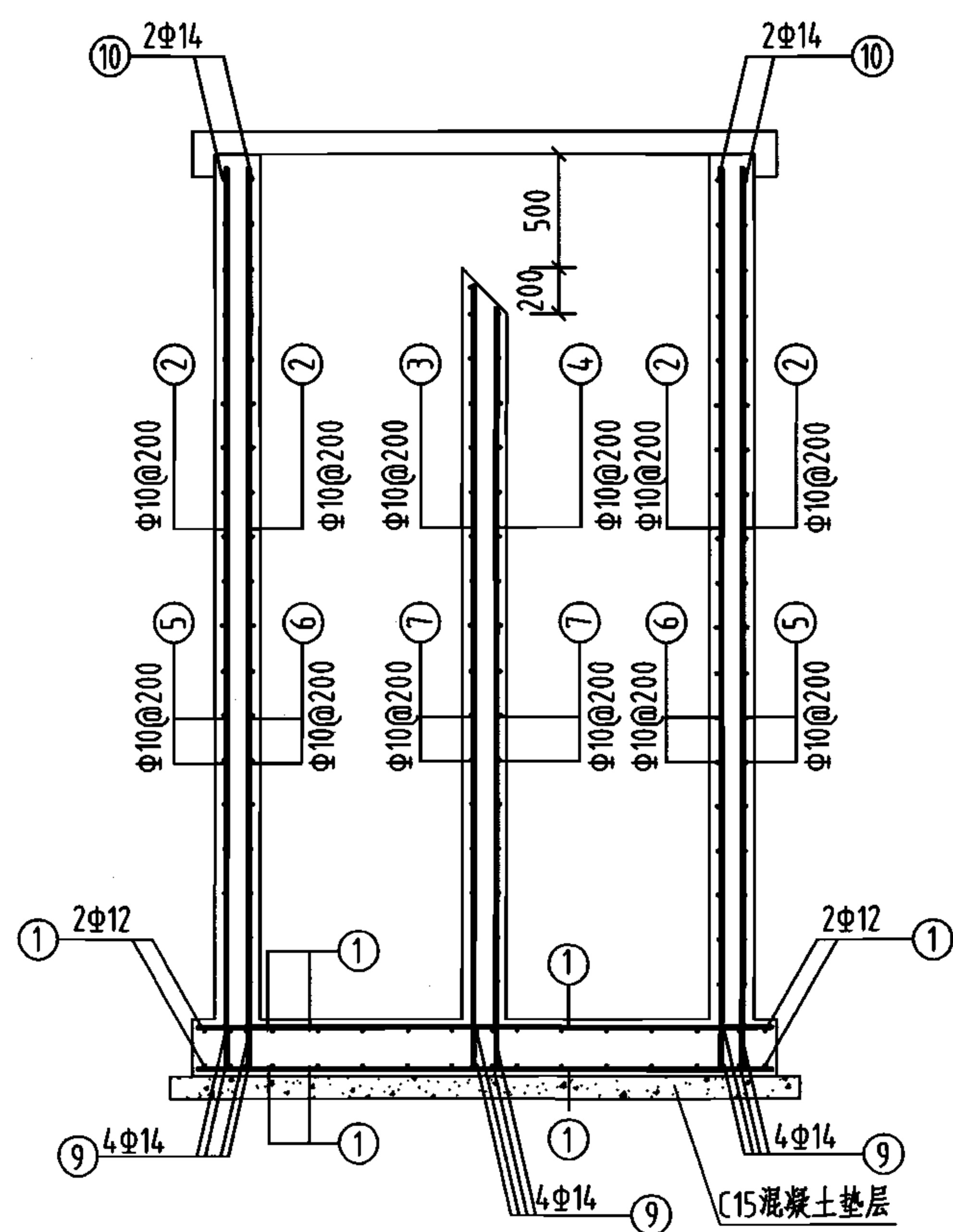
2-2 剖面图
