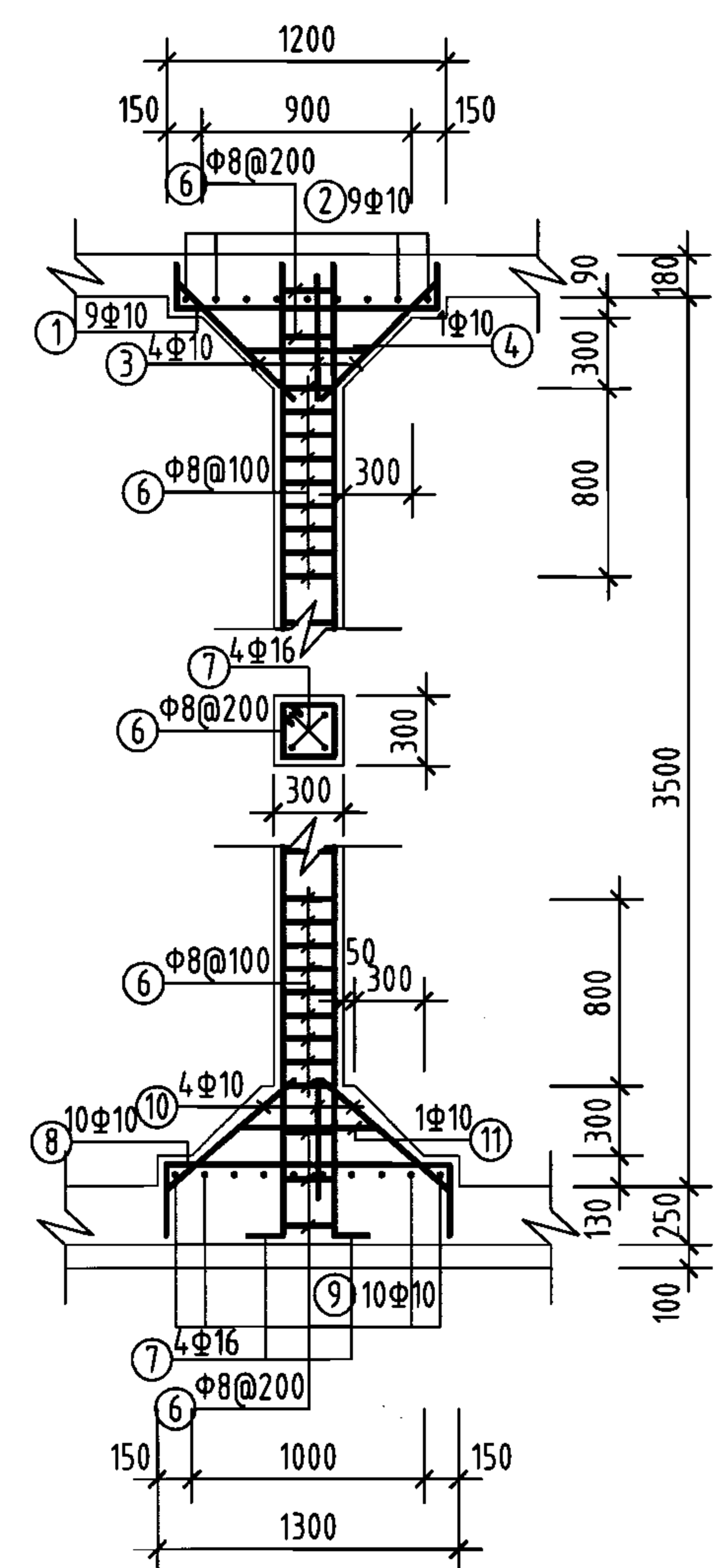
立柱配筋
