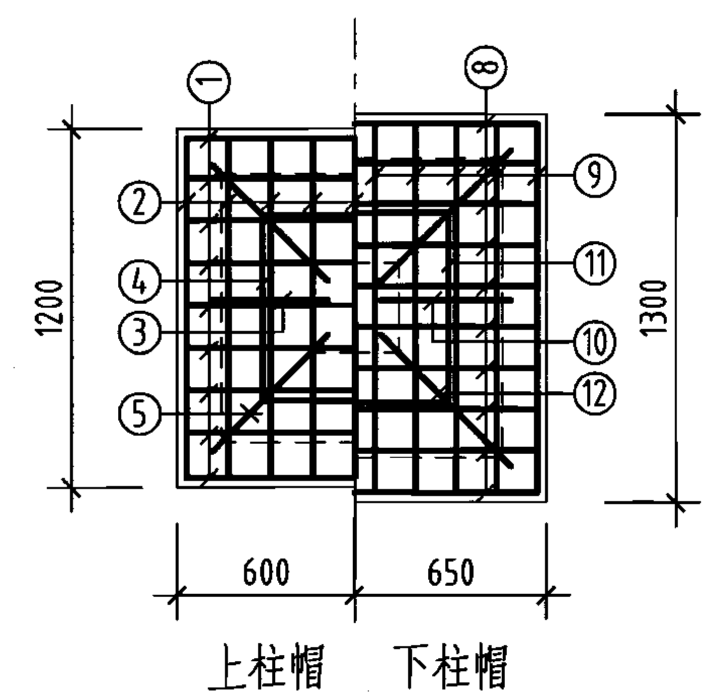
柱帽配筋
