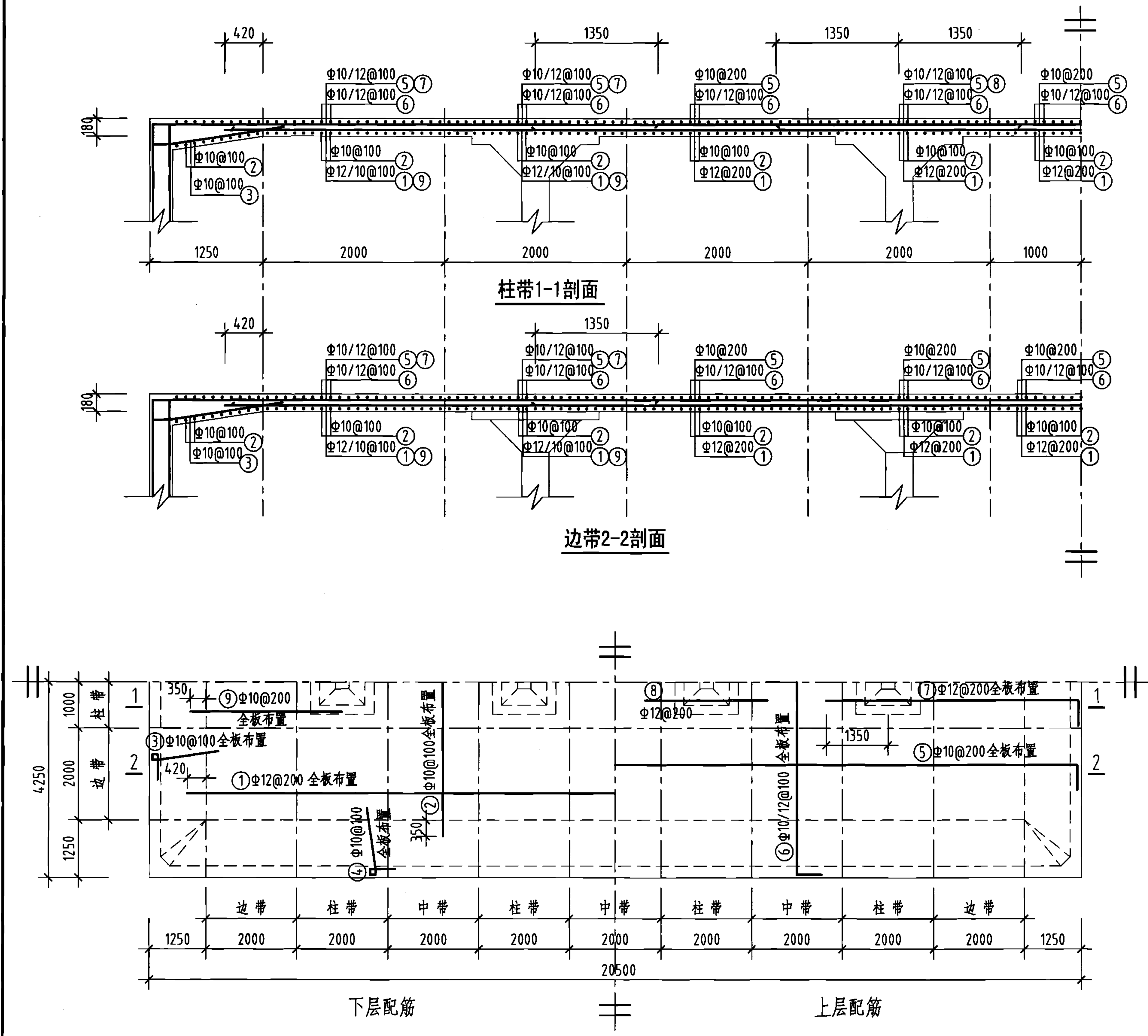
顶板平面配筋图
