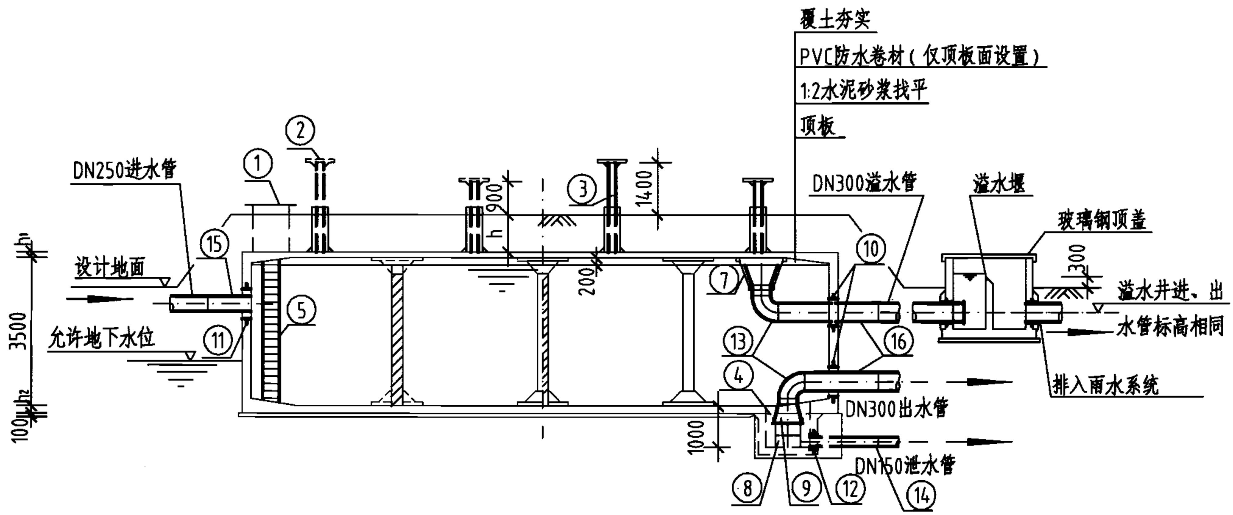
1-1剖面图
