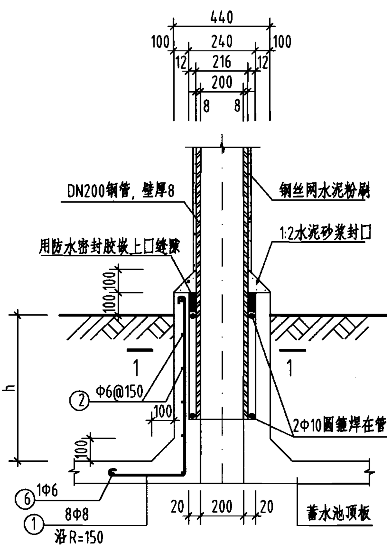
通风管孔钢筋布置图
