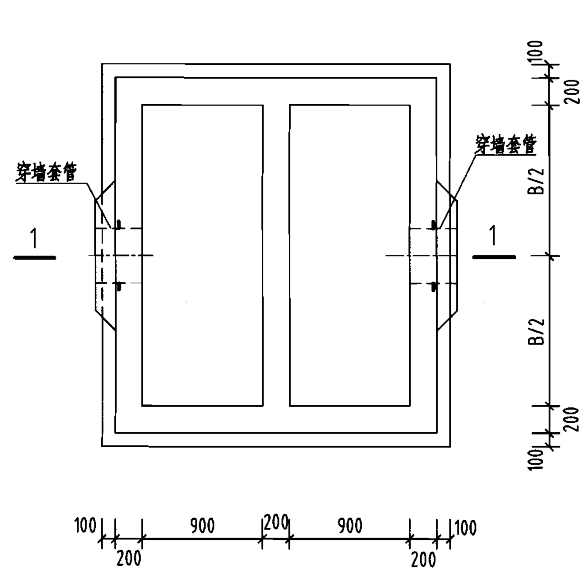
平面布置图
