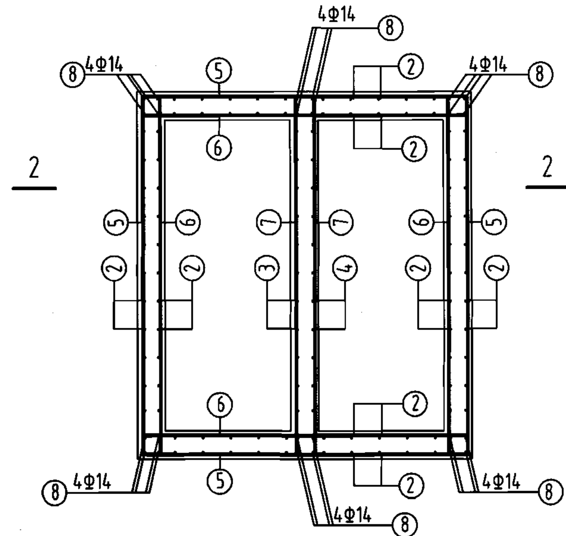
池壁配筋
