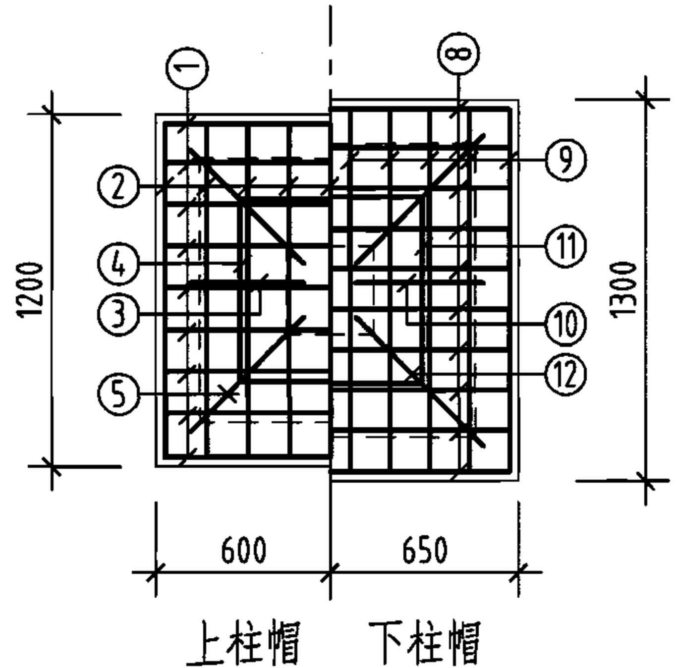
柱帽配筋
