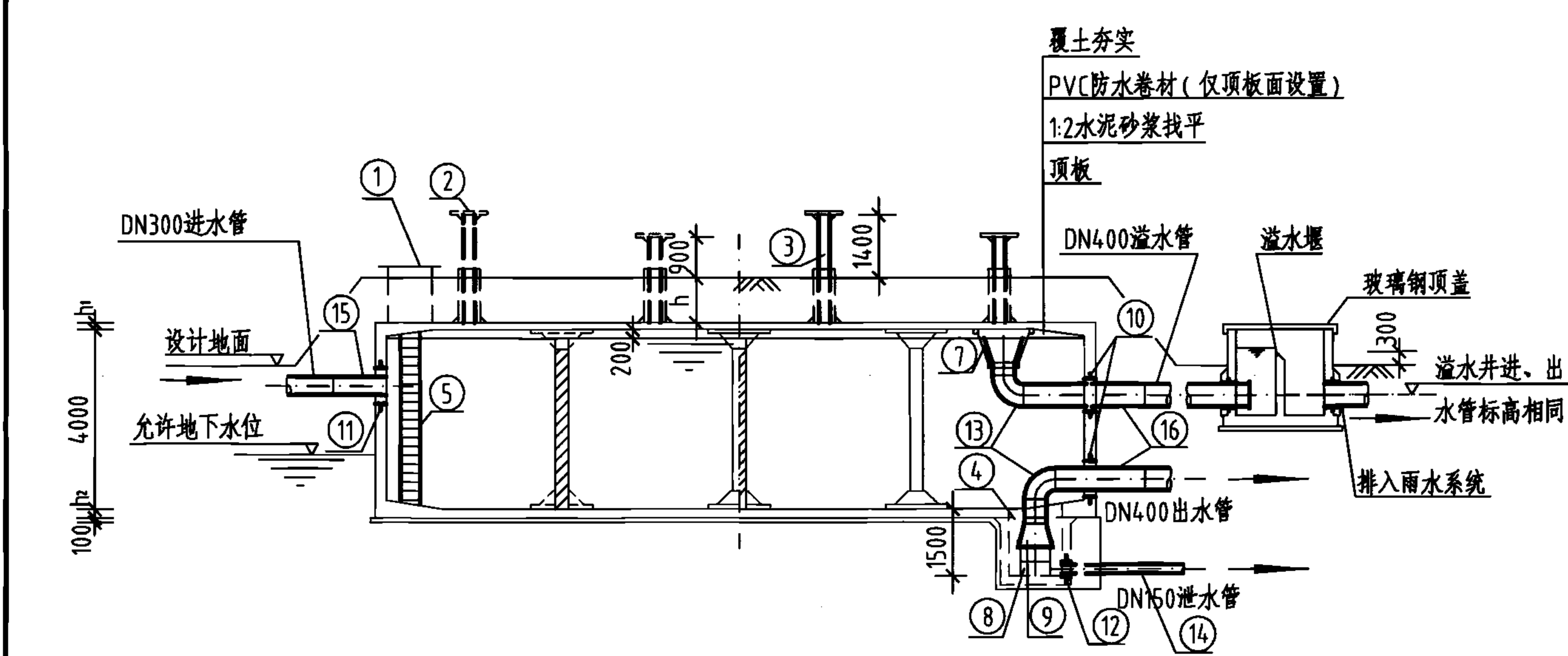
1-1剖面图
