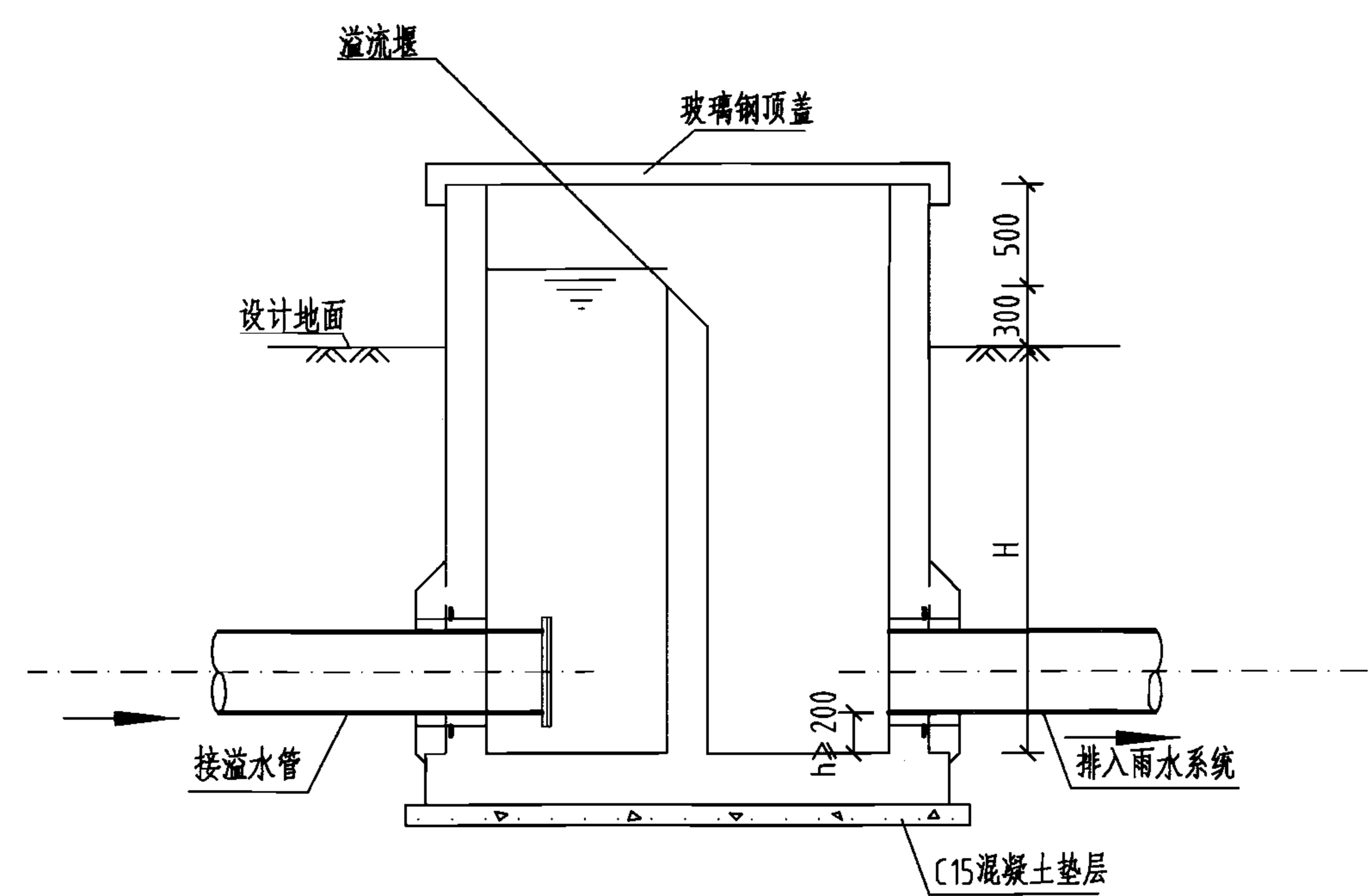
2-2剖面图
