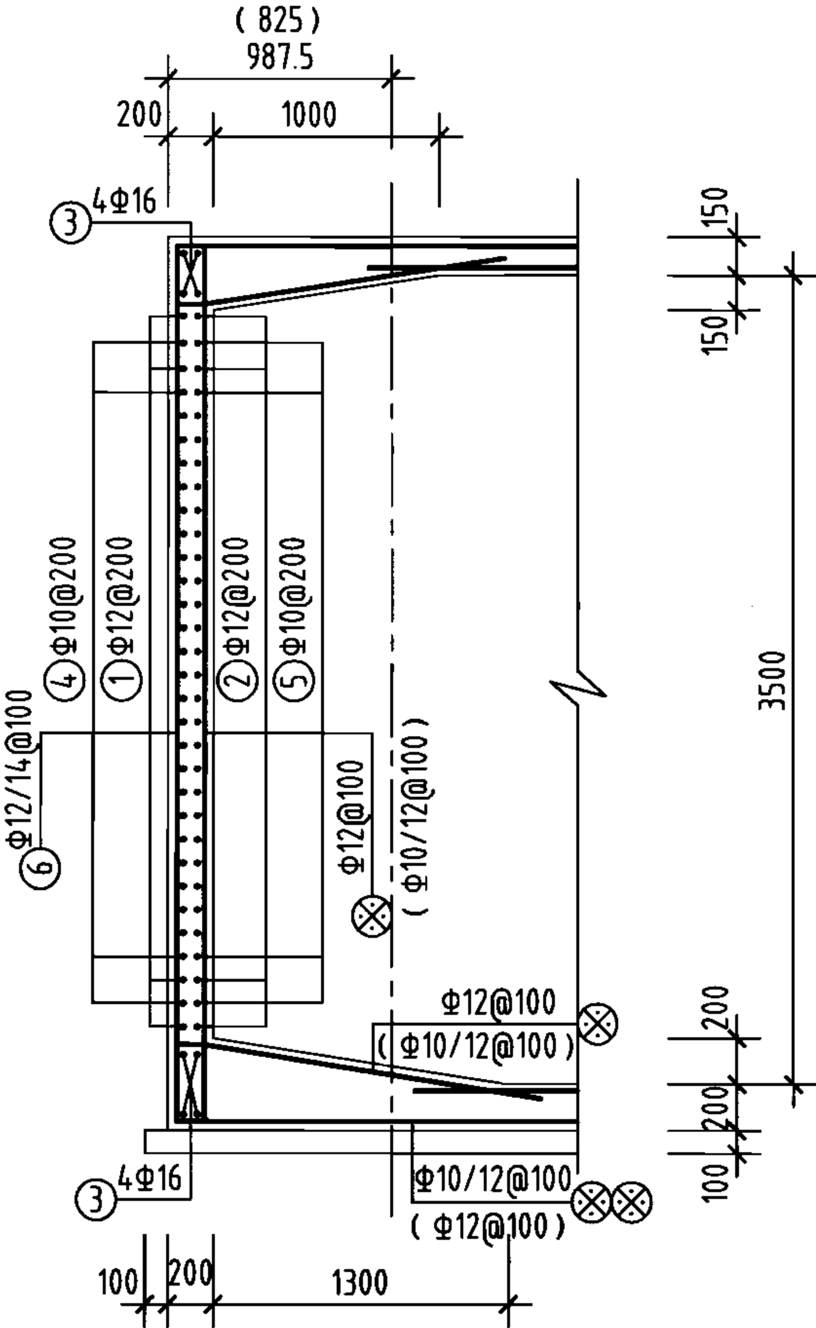
1-1剖面 (1'-1'剖面)
