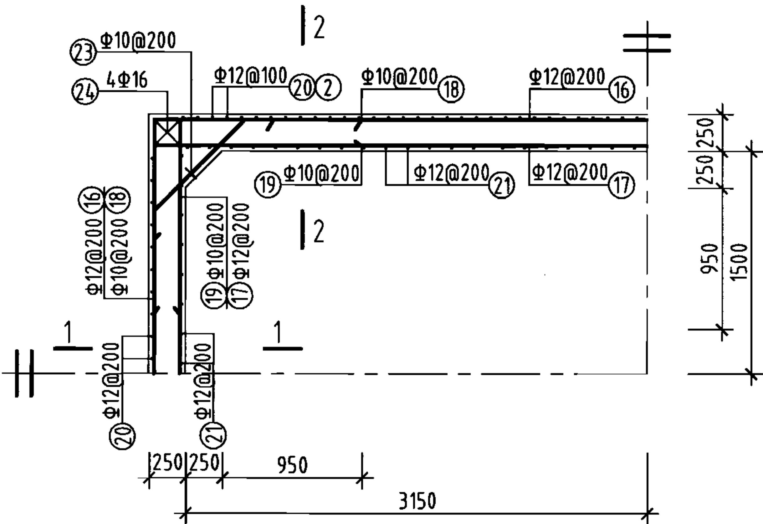
池壁平面配筋图
