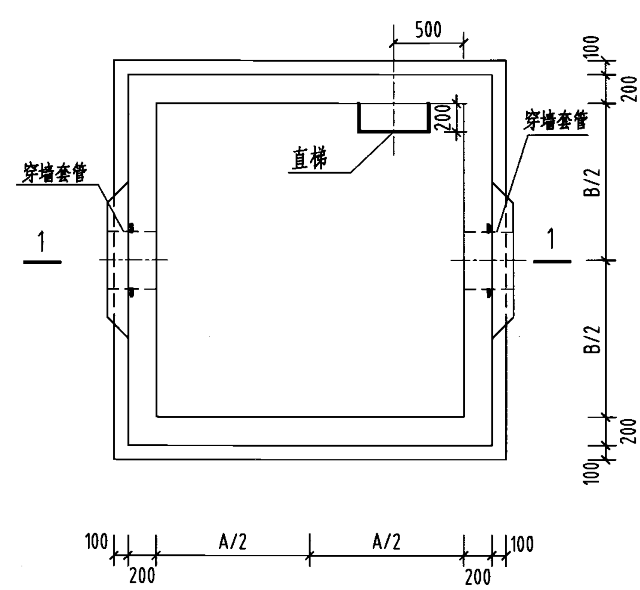
平面布置图
