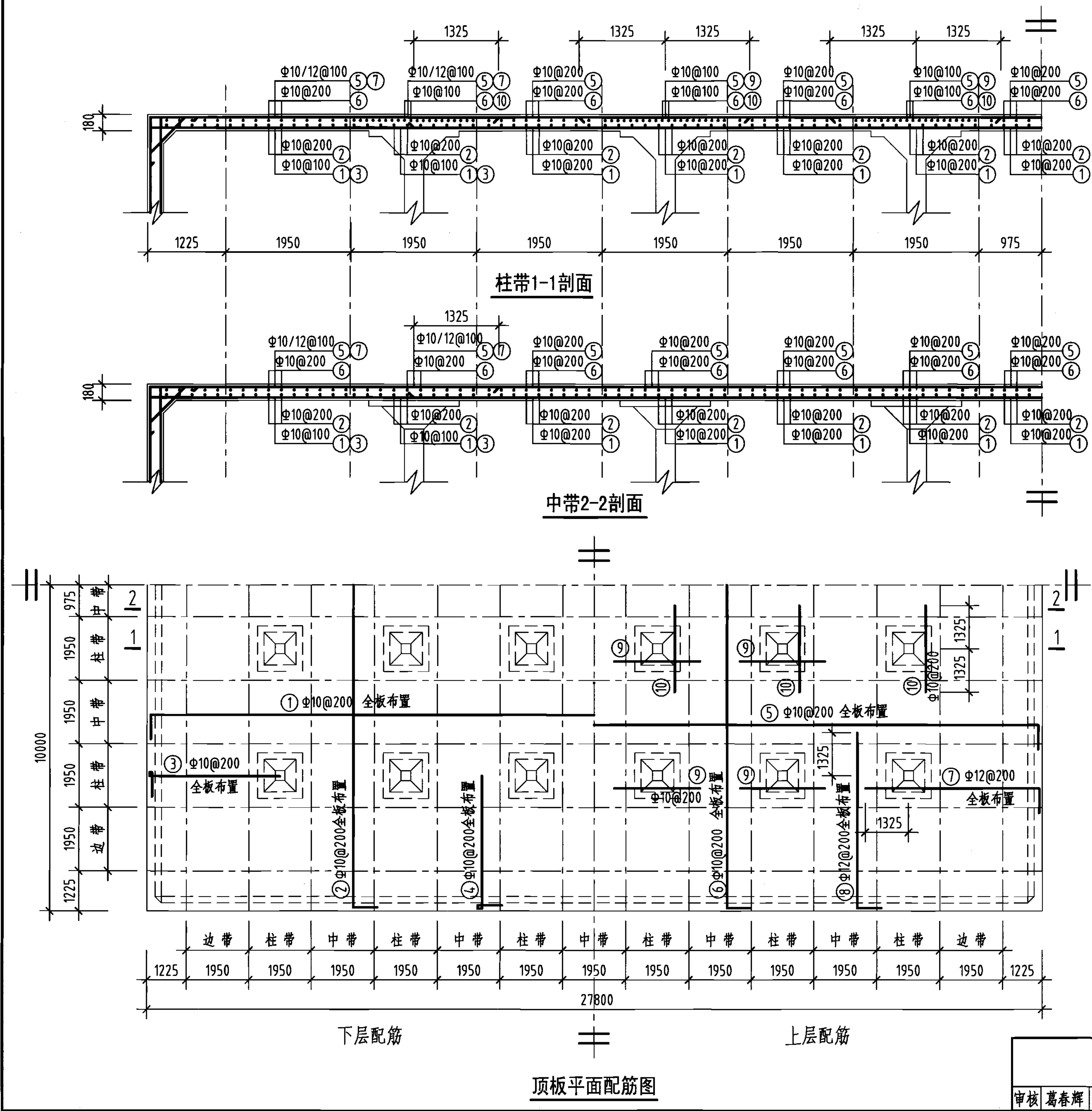
2000m³矩形蓄水池顶板配筋图 (池顶覆土500mm)
