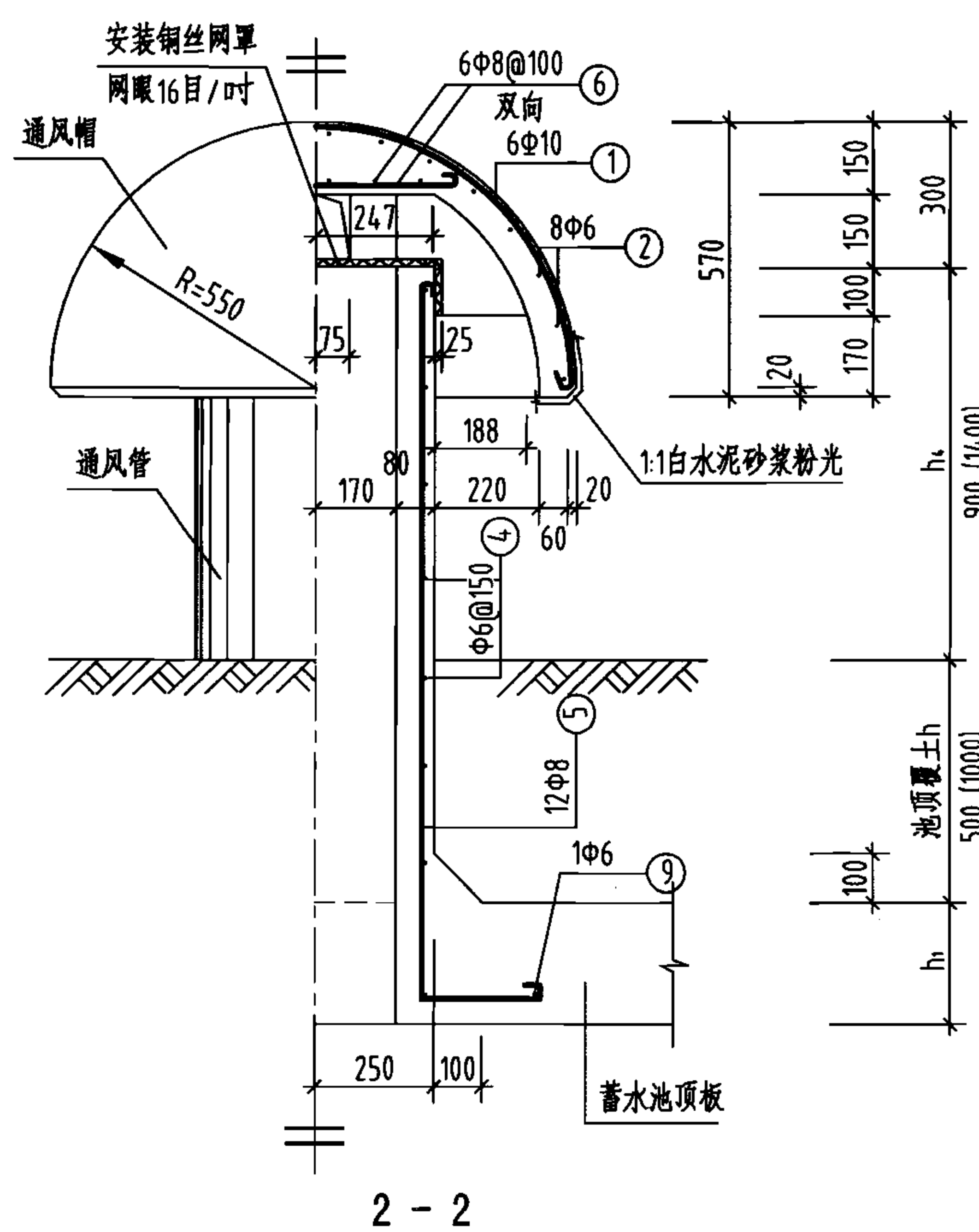
(B1型:池顶覆土为500, B2型:池顶覆土为1000)
