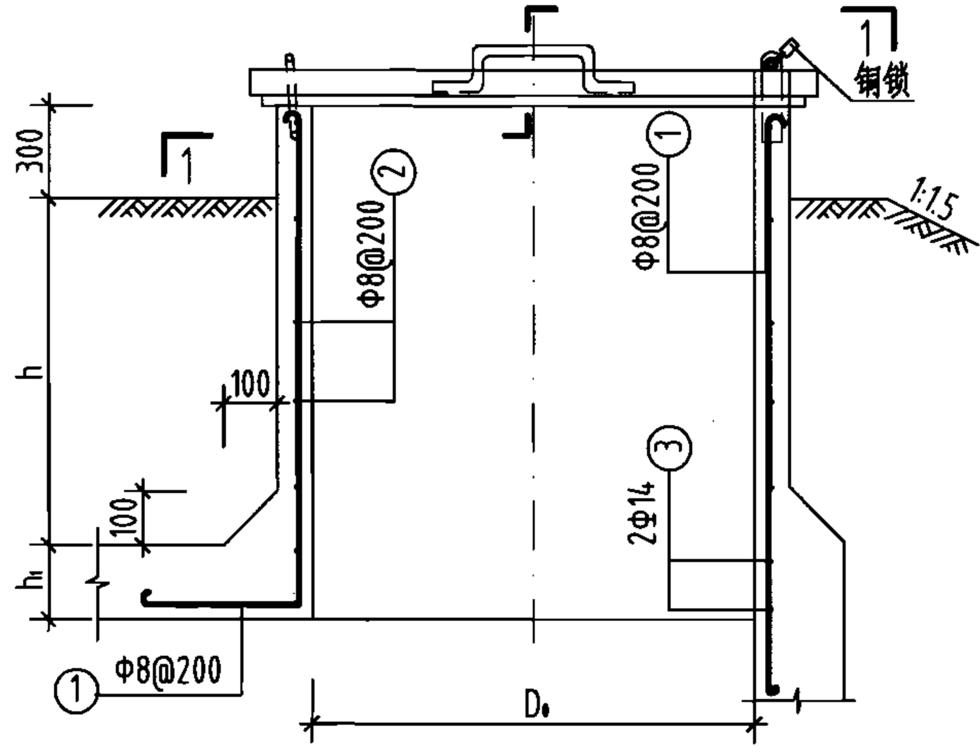
检修孔钢筋布置图
