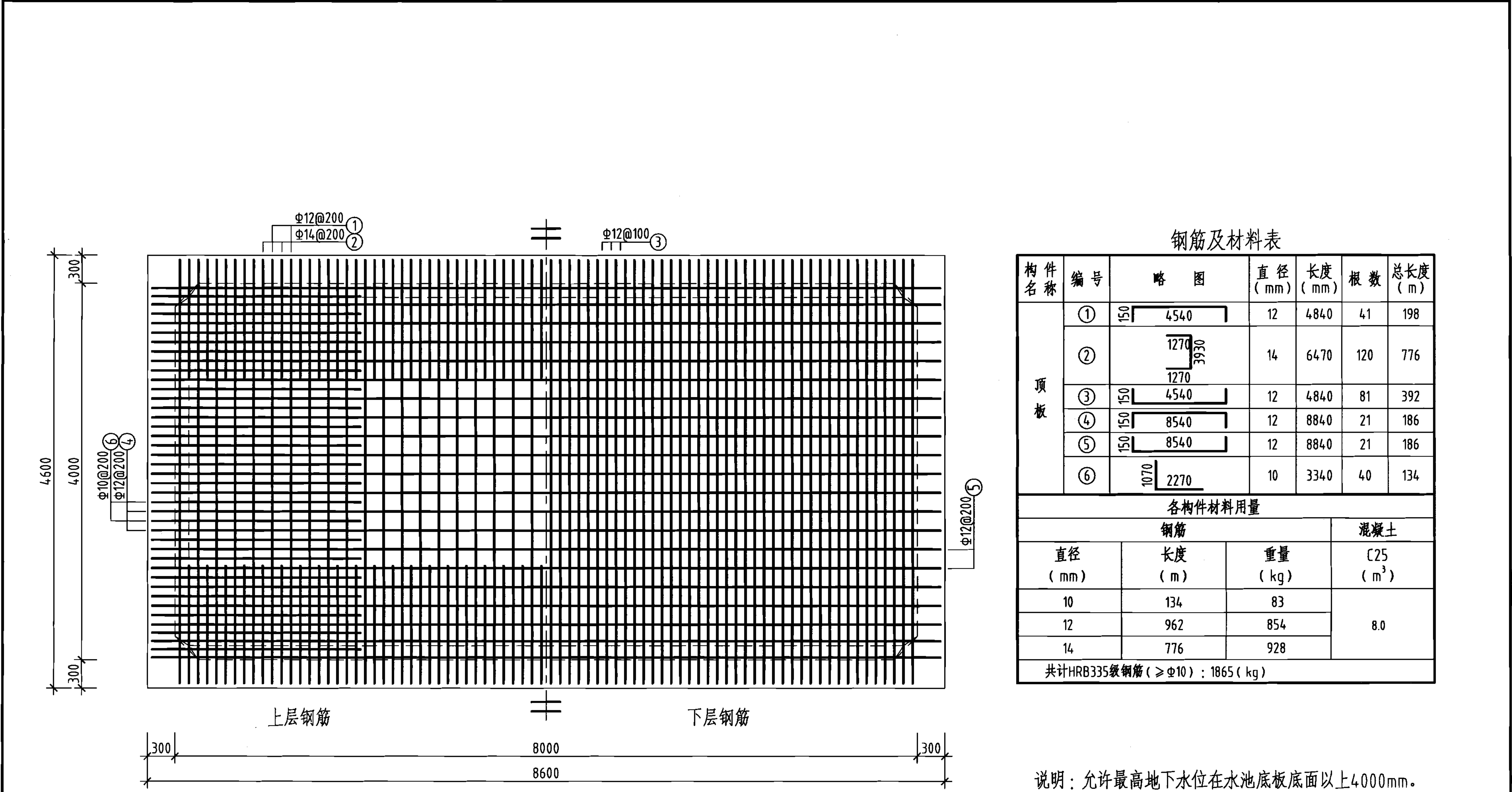
池顶板配筋图
