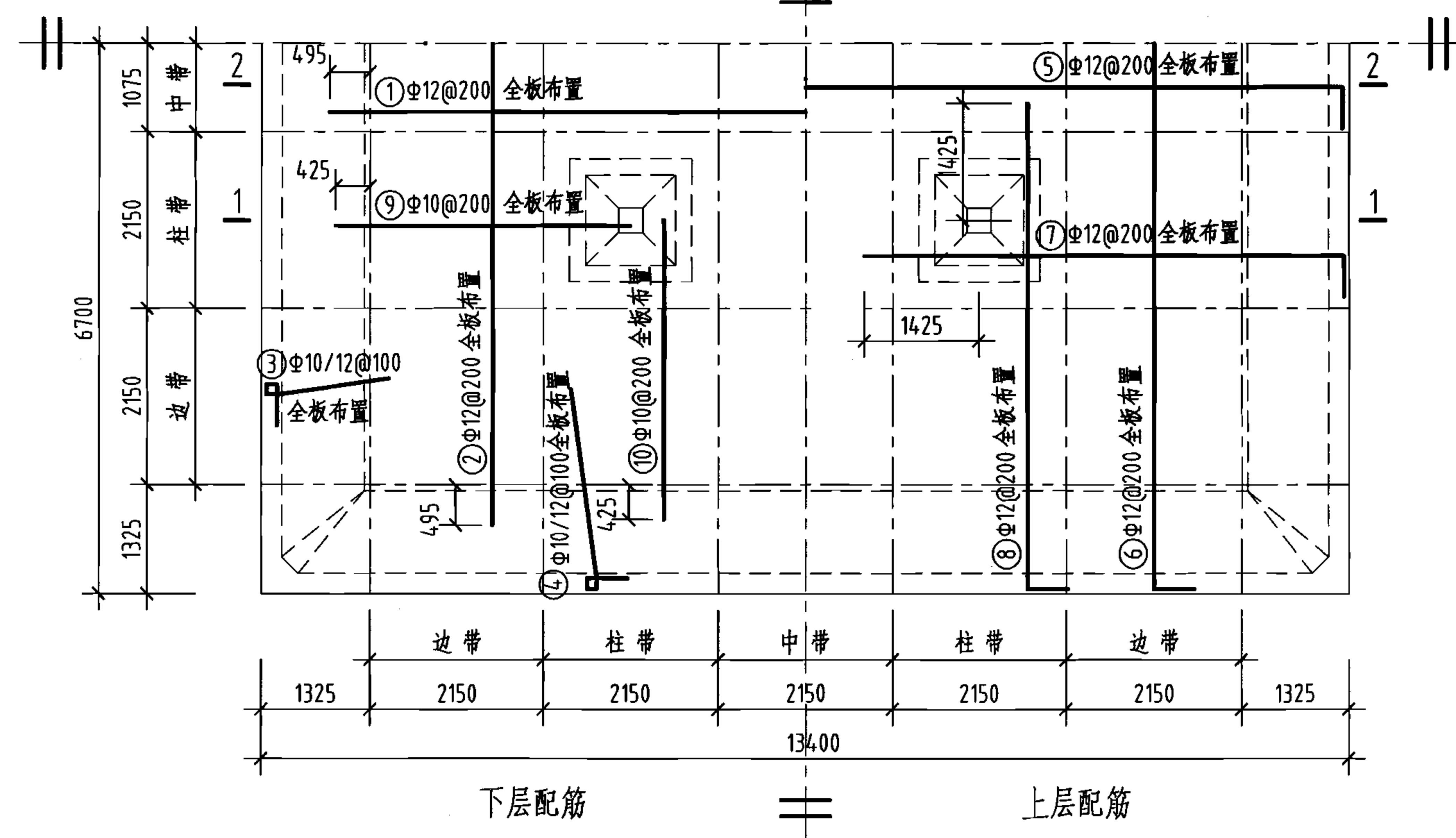
顶板平面配筋图
