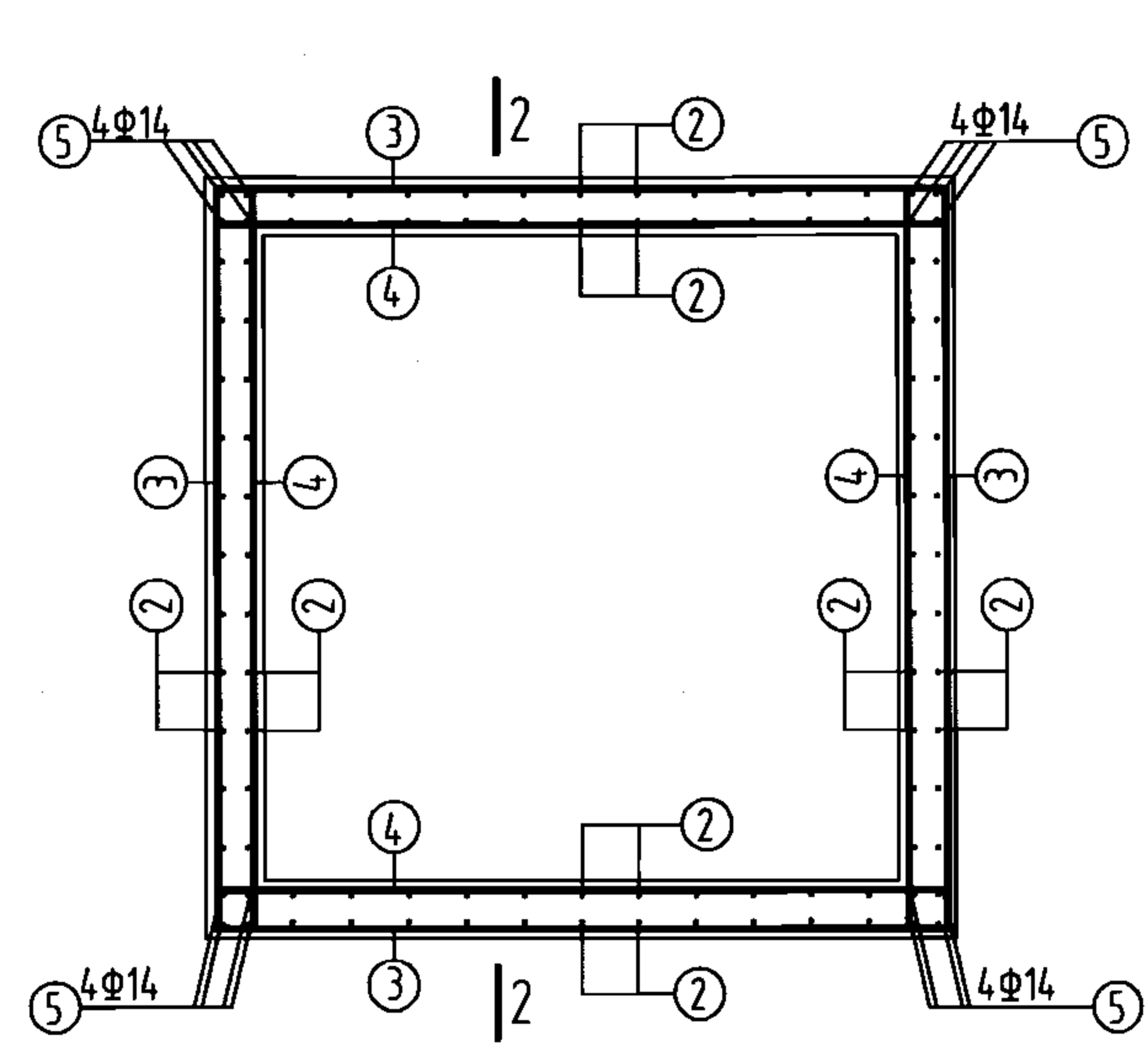
池壁配筋
