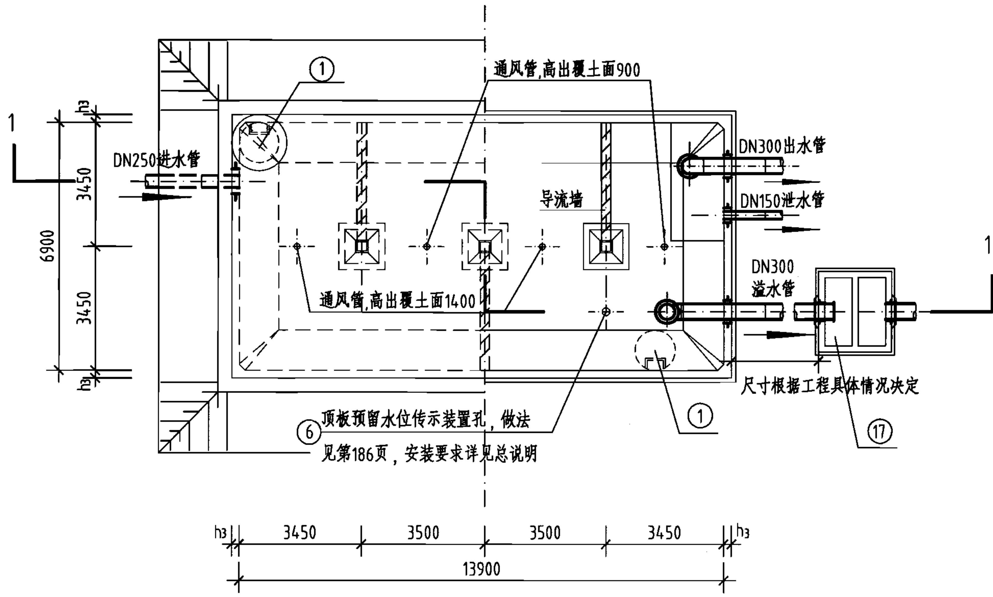
平面图
